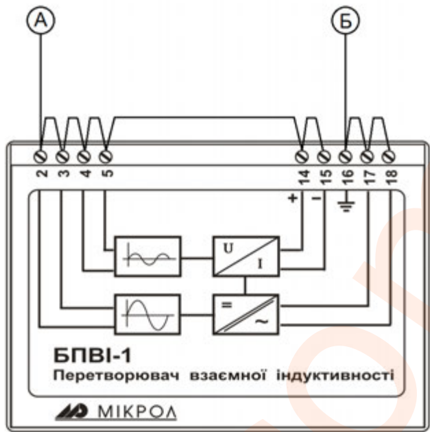
Рисунок А.1 - Схема проверки сопротивления изоляции
