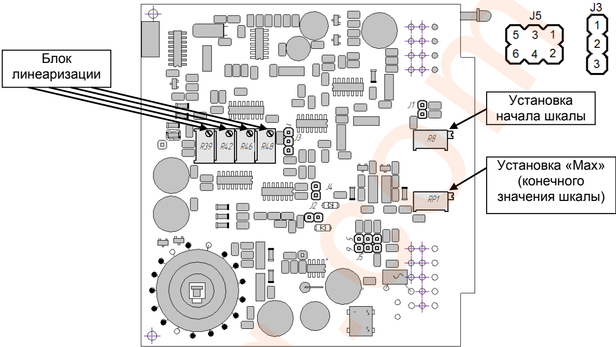
Рисунок 5.1.1 - Схема расположения органов регулирования и элементов настройки БПВ1-10
