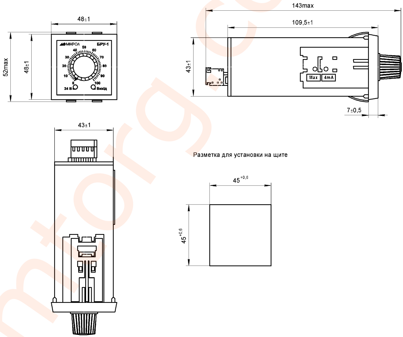
Рисунок 1- Габаритные и установочные размеры блока ручного управления БРУ-1
