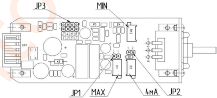
Рисунок 2- Расположение блоков перемычек и органов регулировки выходного сигнала внутри блока ручного управления БРУ-1
