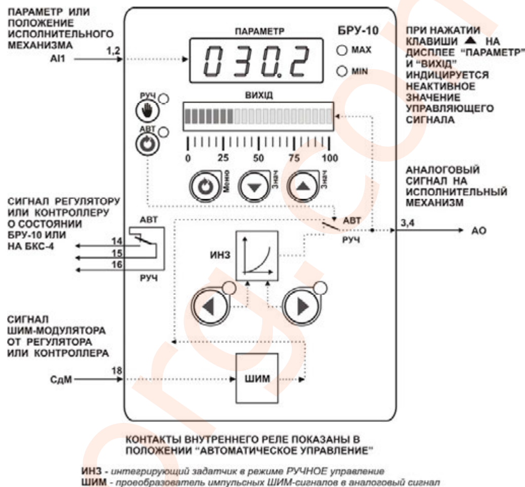
Рисунок 7.6.1 - Блок-схема режима 5
