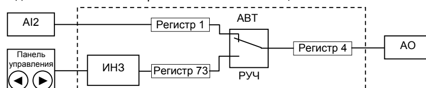
Рисунок 7.12.2 - Функциональная схема балансировки режима 11
