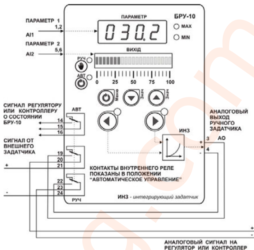
Рисунок 7.1.1 - Блок-схема режима 0
