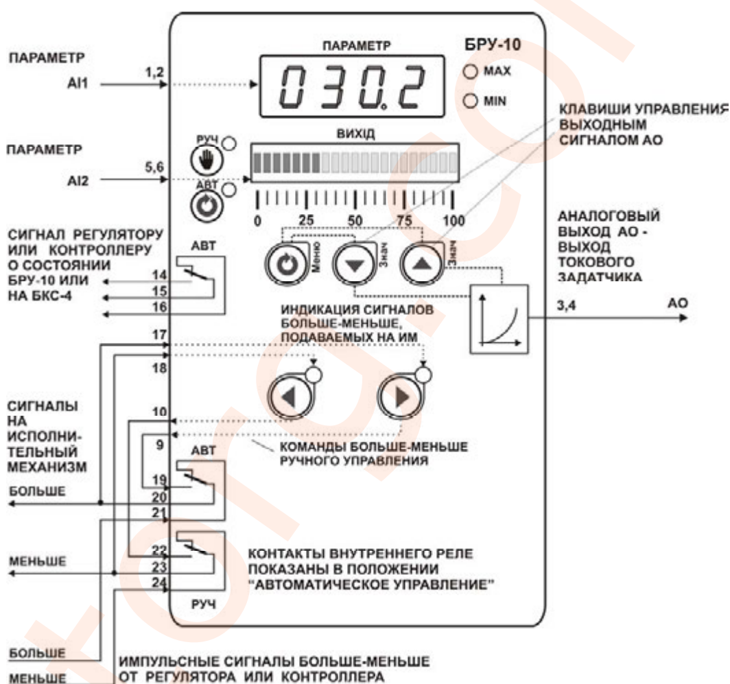
Рисунок 7.9.1 - Блок-схема режима 8
