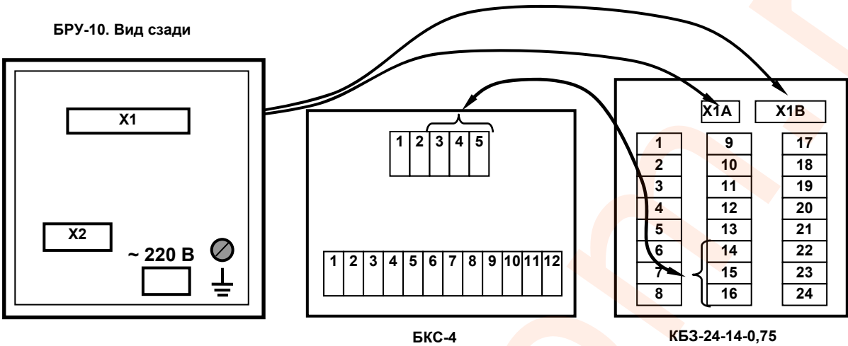
Рисунок Б.1 - Подключение клеммно-блочного соединителя КБЗ-24-14-0,75 к блоку ручного управления БРУ-10
