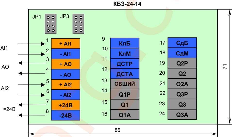
Рисунок Б.1 - Подключение клеммно-блочного соединителя КБЗ-24-14-0,75 к блоку ручного управления БРУ-10
