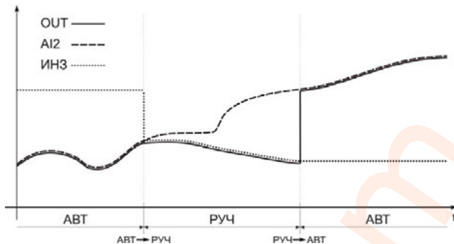
Рисунок 7.3 – График работы балансировок режима 3
