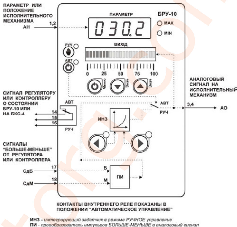
Рисунок 7.10.1 - Блок-схема режима 9
