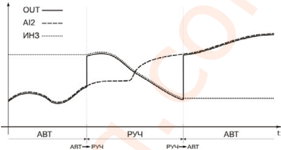
Рисунок 7.1 – График работы балансировок режима 1
