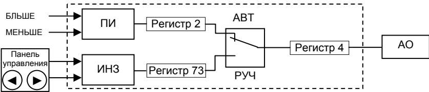
Рисунок 7.5.2 - Функциональная схема балансировок режима 4
