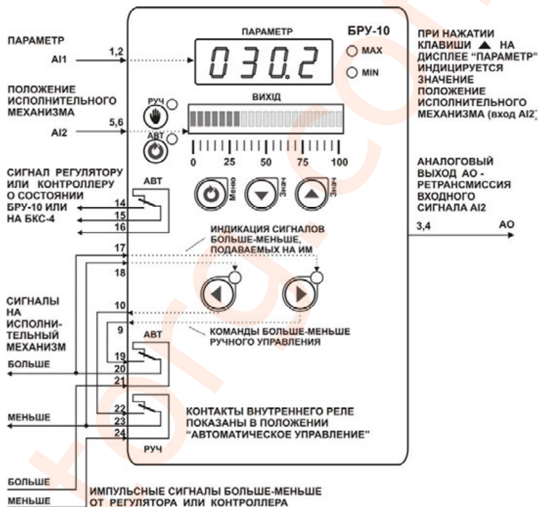
Рисунок 7.4.1 - Блок-схема режима 3
