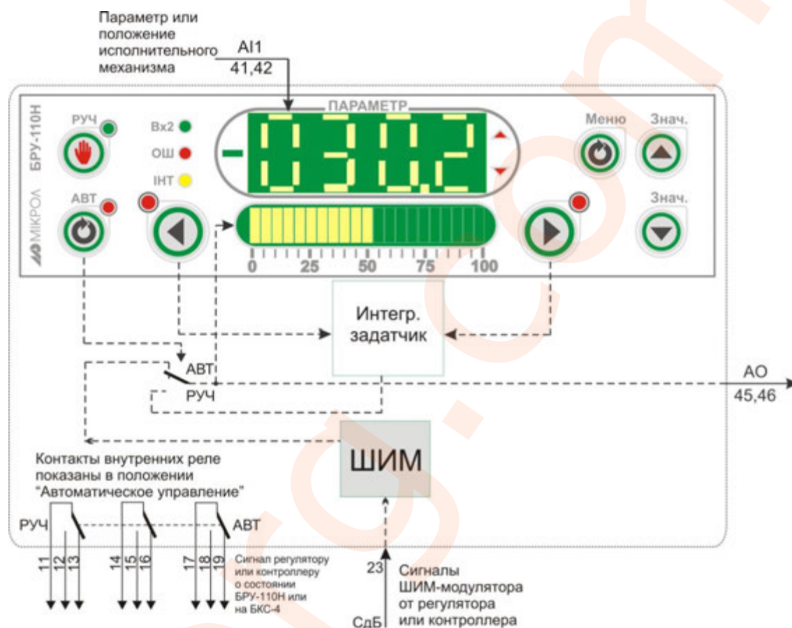
Рисунок 4.14 - Блок-схема режима 5
