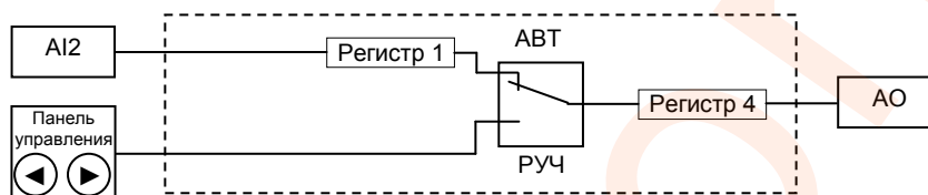
Рисунок 4.9 - Функциональная схема балансировки режима 1
