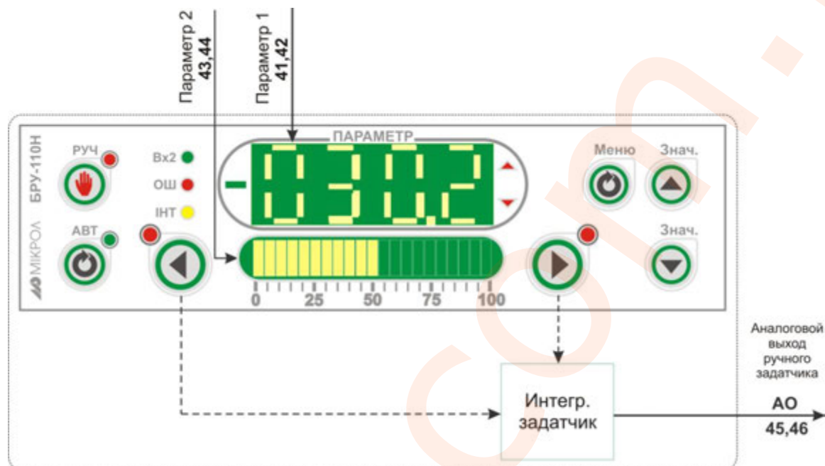
Рисунок 4.7 - Блок-схема режима 0
