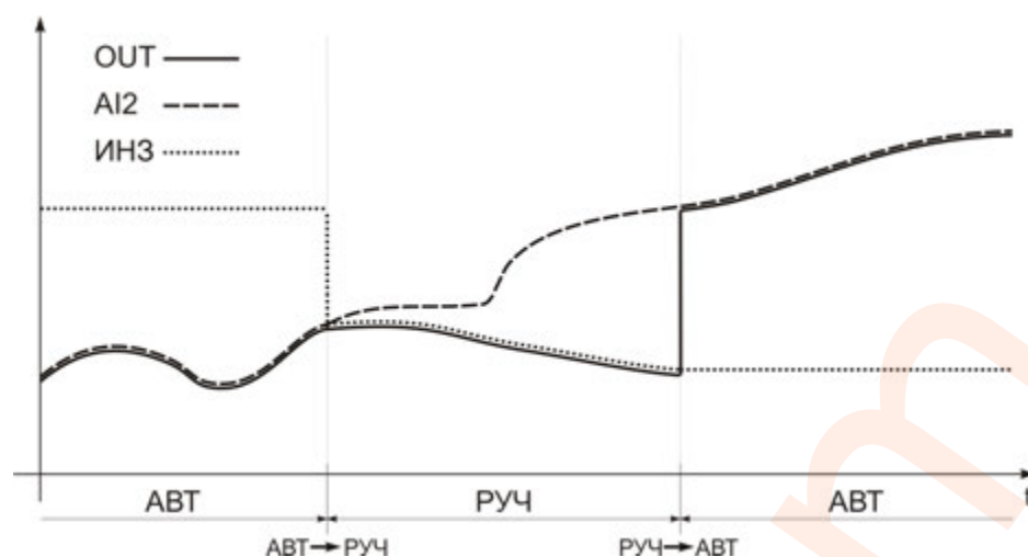
Рисунок 4.5 – График работы балансировок режима 3
