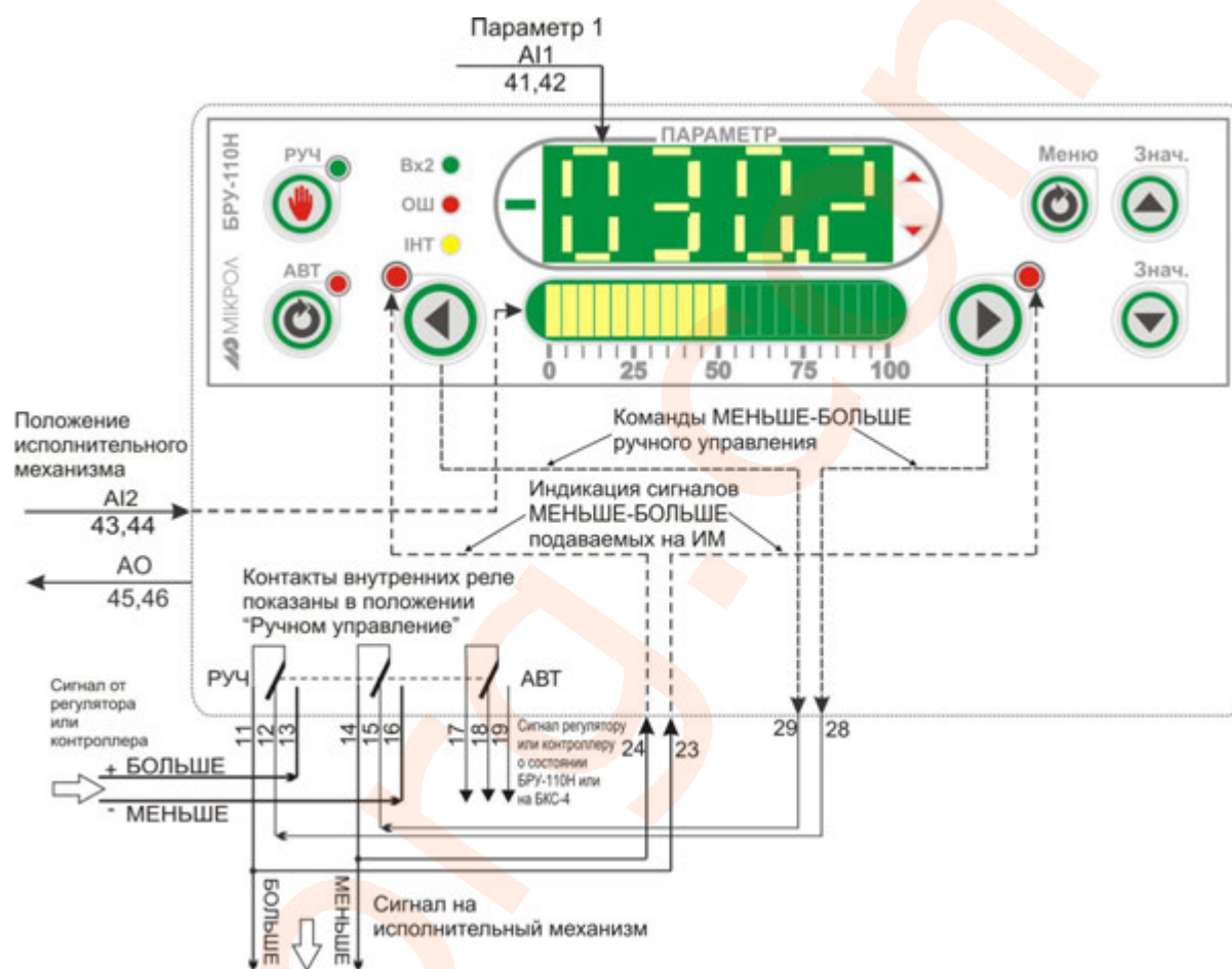
Рисунок 4.11 - Блок-схема режима 3
