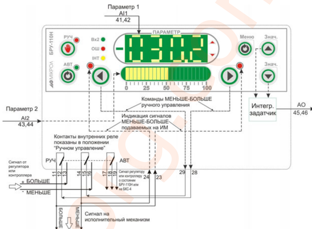
Рисунок 4.17 - Блок-схема режима 7
