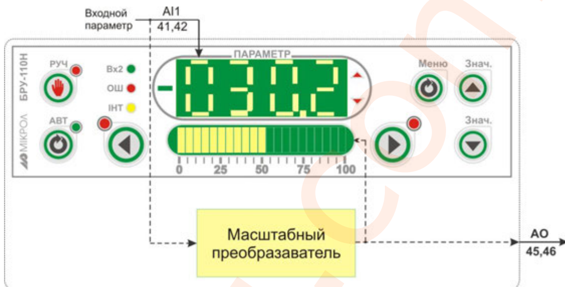
Рисунок 4.16 - Блок-схема режима 6
