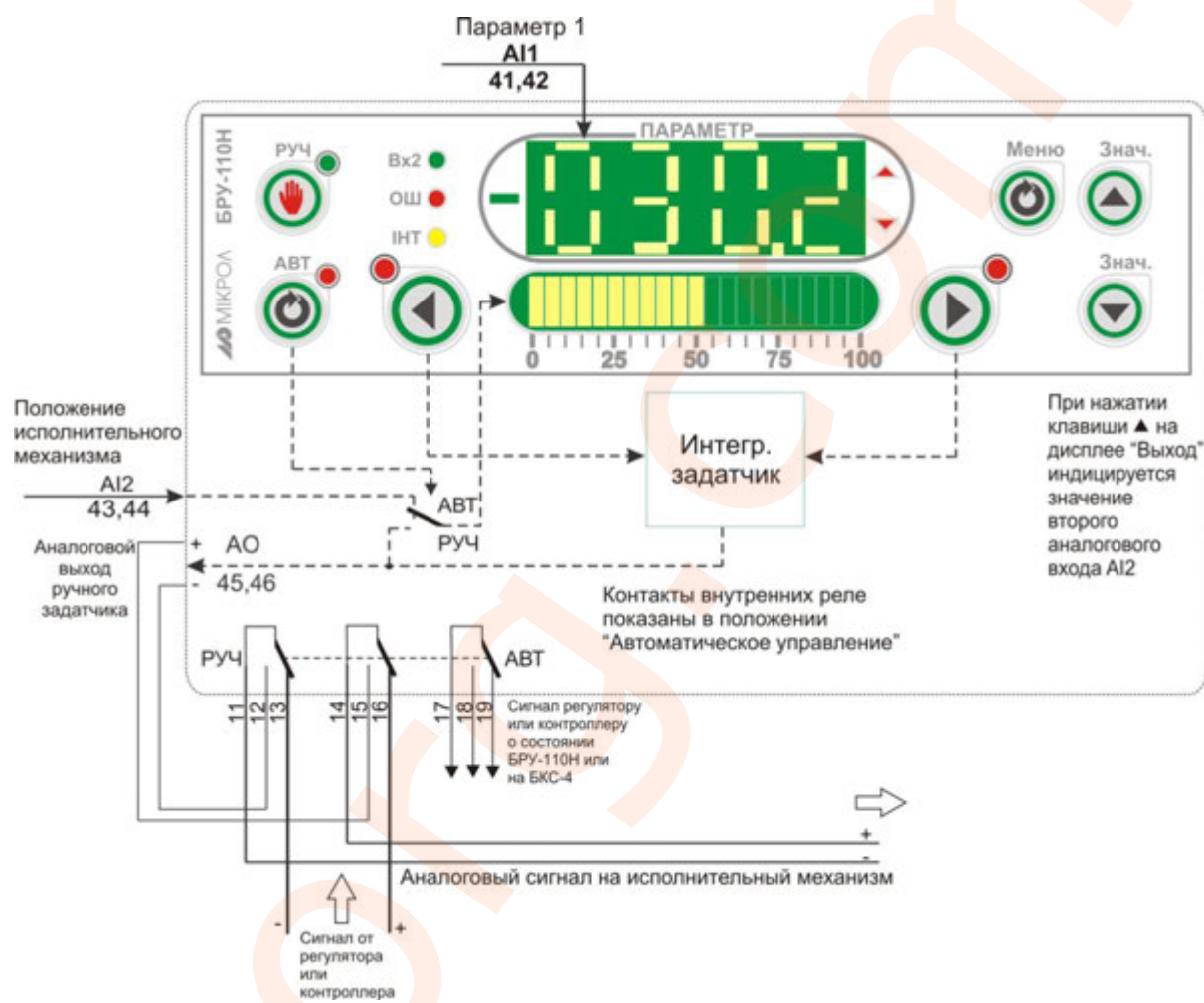
Рисунок 4.8 - Блок-схема режима 1
