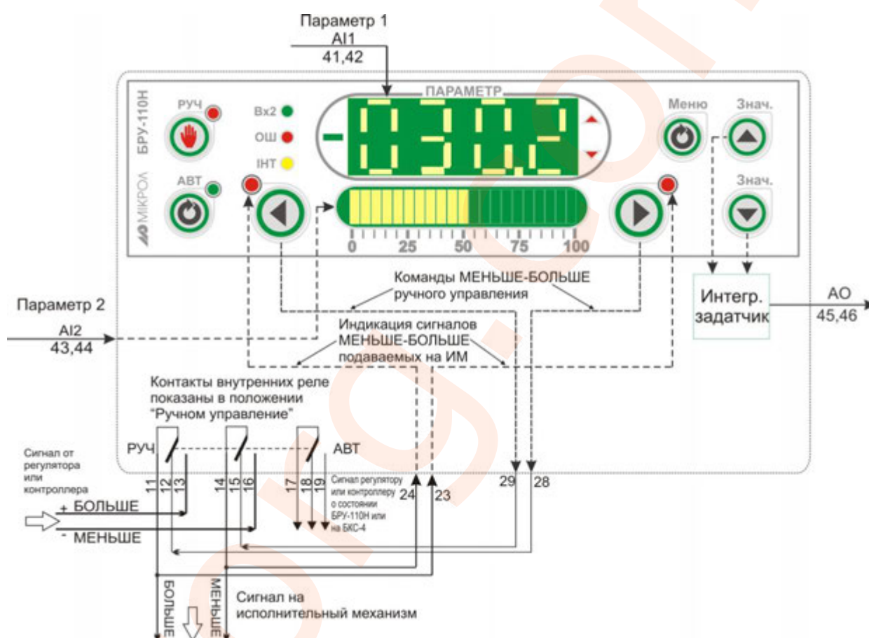
Рисунок 4.18 - Блок-схема режима 8
