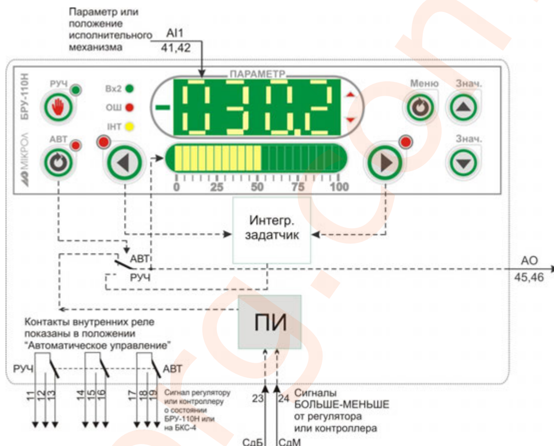
Рисунок 4.19 - Блок-схема режима 9
