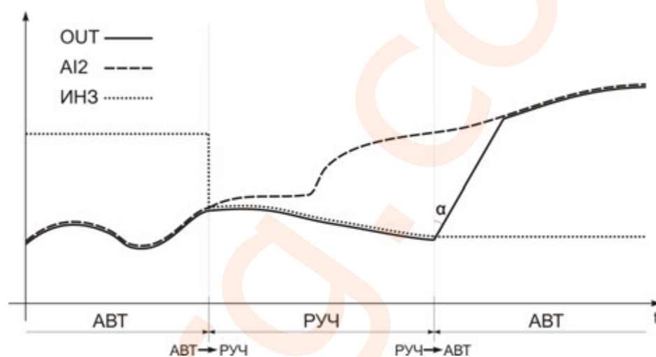
Рисунок 4.6 – График работы балансировок режима 4
