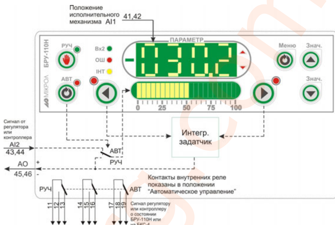
Рисунок 4.10 - Блок-схема режима 2
