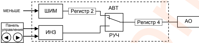
Рисунок 4.15 - Функциональная схема балансировок режима 5
