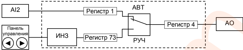
Рисунок 4.24 - Функциональная схема балансировок режима 11
