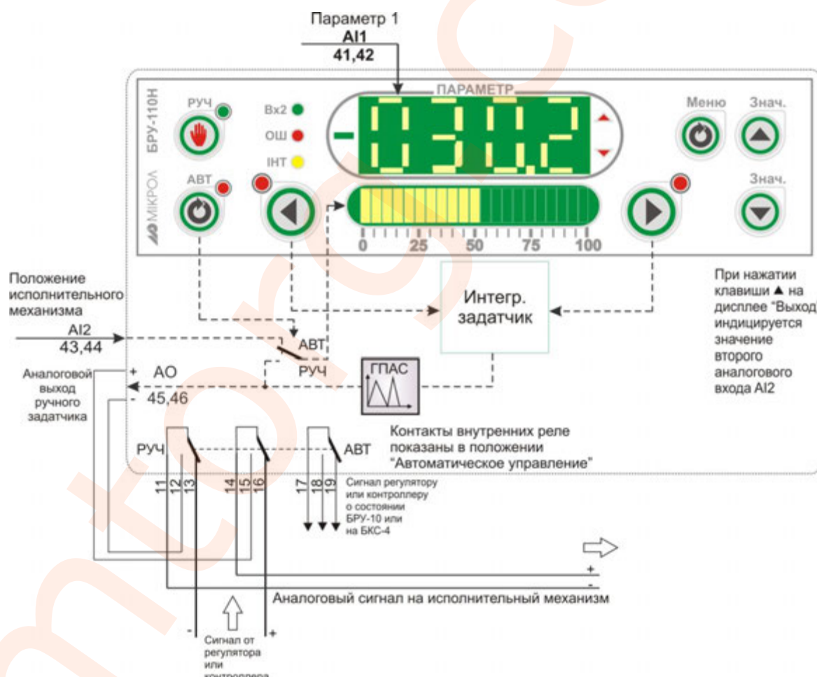
Рисунок 4.22 - Блок-схема режима 10
