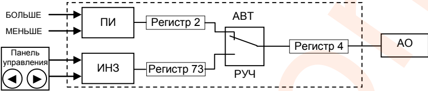
Рисунок 4.13 - Функциональная схема балансировок режима 4
