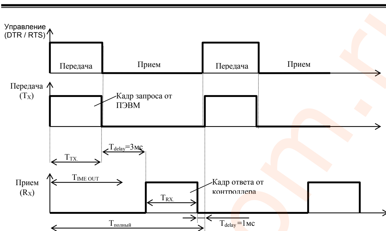
Рисунок В.1 - Временные диаграммы управления передачей и приемом блока интерфейсов БПИ-485 (БПИ-52)
