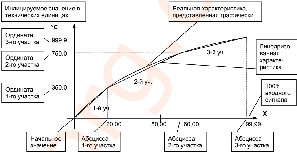
Пример 1. Линеаризация сигнала, подаваемого на вход AI, представленная графически (кривой)
