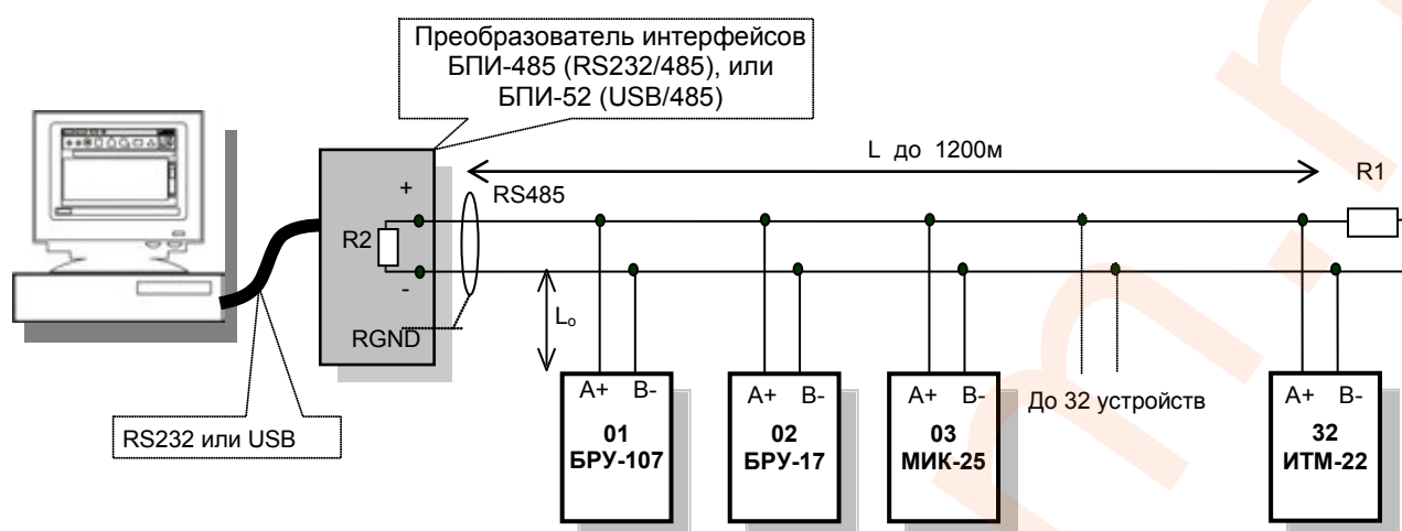
Рисунок Б.6 - Организация интерфейсной связи между компьютером и блоками или контролерами
