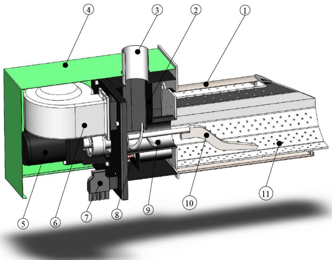
Рисунок 1 - Основные компоненты горелки.
