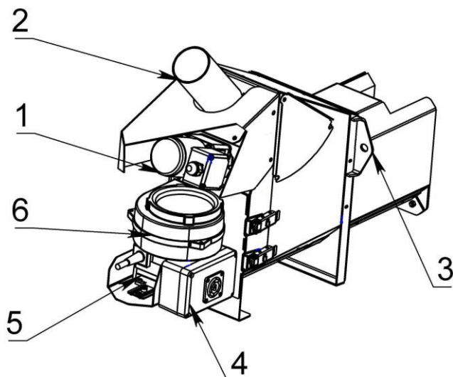
Рис. 4 – Устройство горелки
