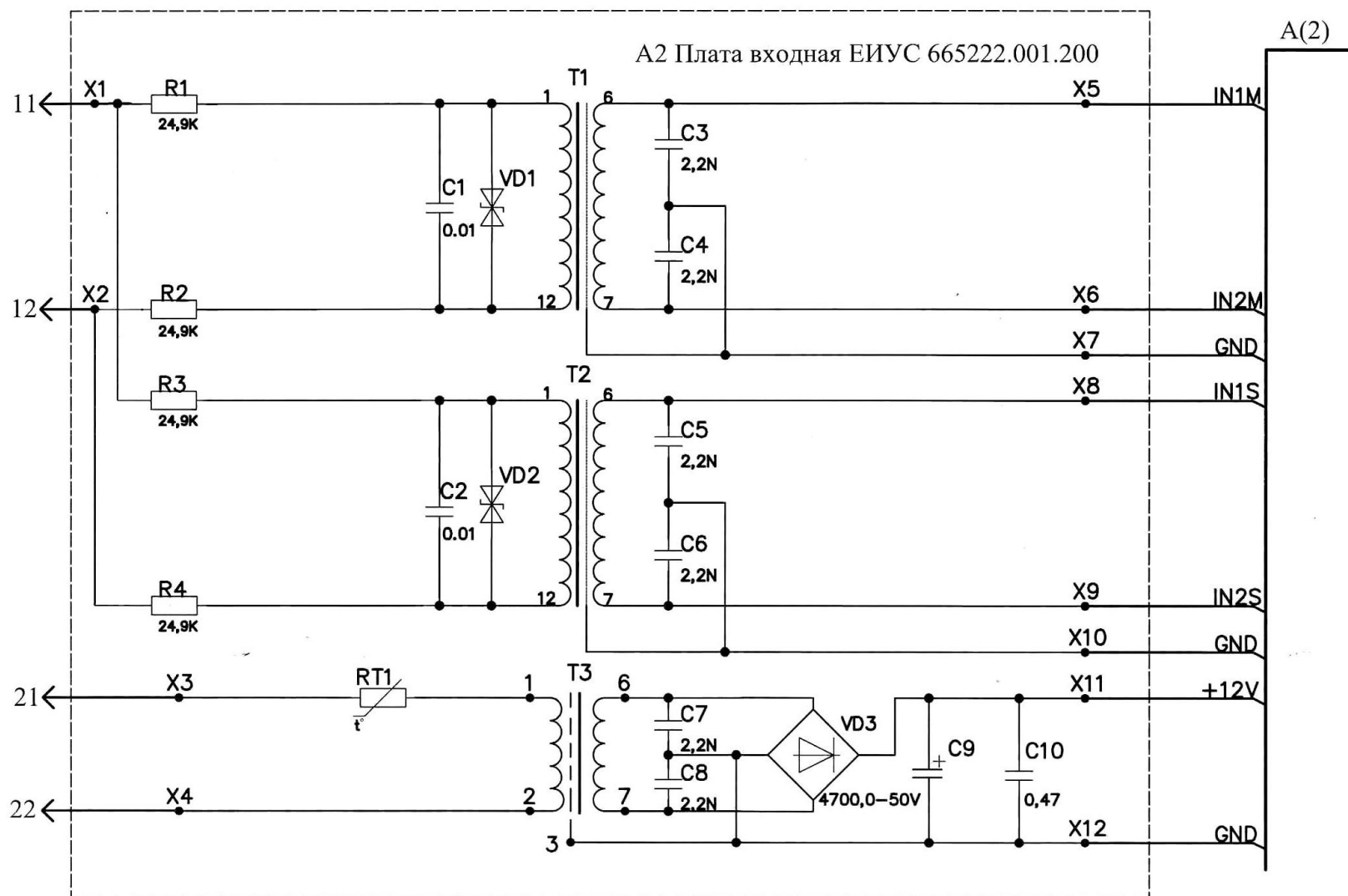
Б1. Схема электрическая принципиальная устройства безопасного контроля напряжения УБKN1 плата А2
