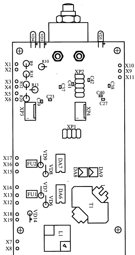
Плата А1
