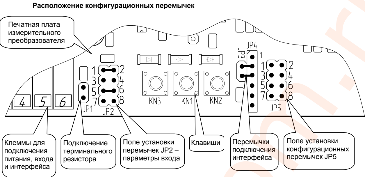
Рисунок 6.2 - Расположение конфигурационных перемычек на плате ИТМ-1-01-31 и ИТМ-1-01-41
