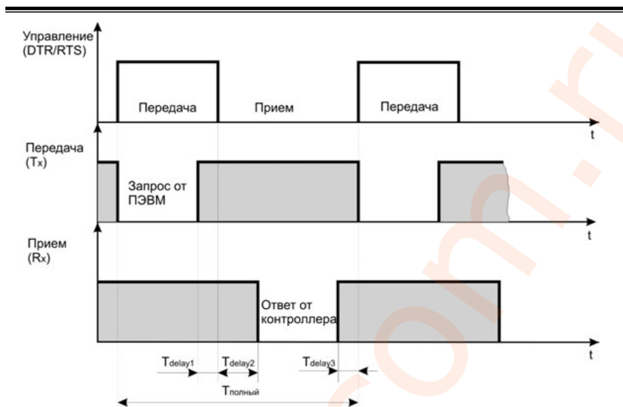
Рисунок 7.1 - Временные диаграммы управления передачей и приемом блока интерфейсов БПИ-485
