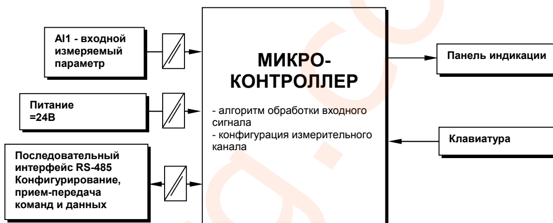
Рисунок 5.3 - Структурная схема индикаторов ИТМ-1-01-31 и ИТМ-1-01-41
