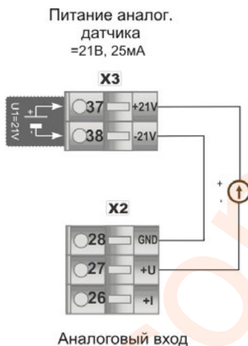
Рисунок Б.2 - Подключение к индикатору ИТМ-110 аналоговых датчиков с пассивными выходами
