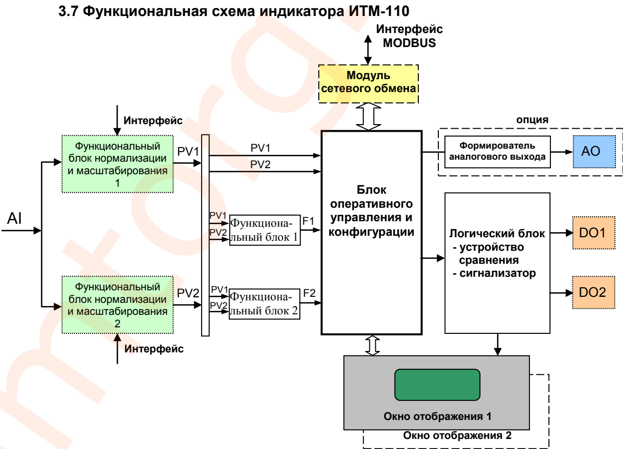
Рисунок 3.3 - Функциональная схема индикатора ИТМ-110
