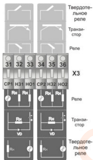
Рисунок Б.3 - Подключение нагрузок при использовании транзисторных выходов
