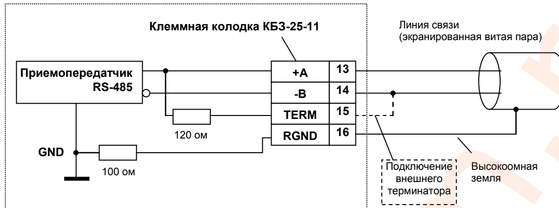
Рисунок Б.18 – Рекомендуемая схема подключения интерфейса RS-485 с помощью KB3-25-11
