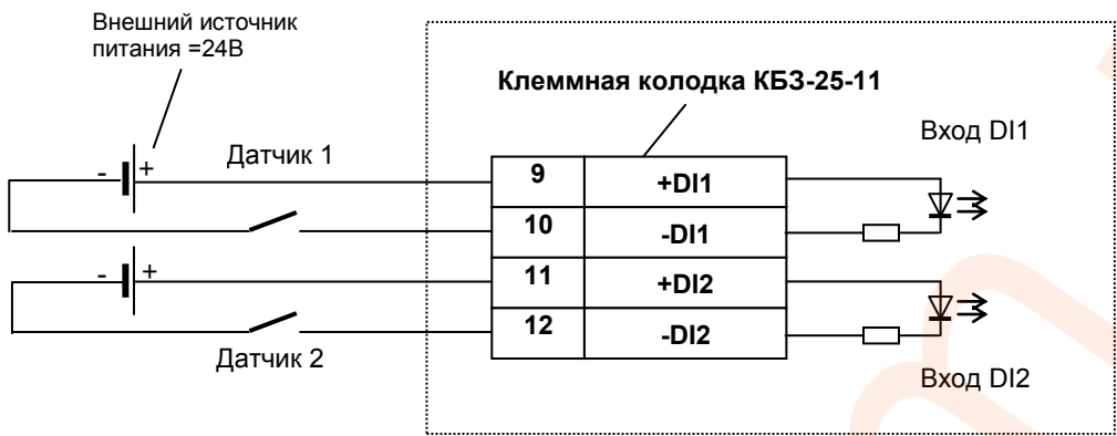
Рисунок Б.20 – Подключение дискретных входов (датчиков) к индикатору с помощью КБ3-25-11
