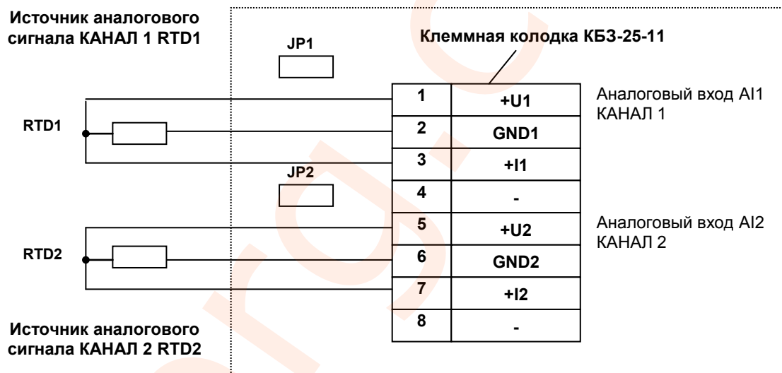
Рисунок Б.7 – Подключение датчиков температуры типа ТСМ, ТСР к аналоговым входам индикатора ИТМ-22У(20У)
