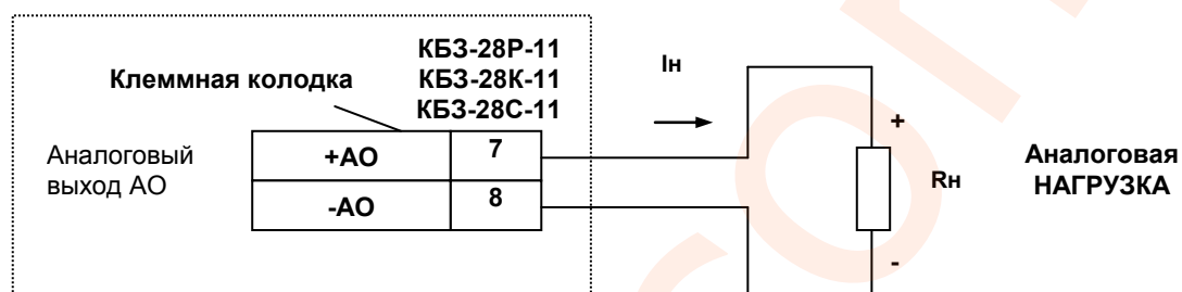
Рисунок Б.11 – Подключение аналоговых нагрузок с помощью КБ3-28Р-11, КБ3-28К-11, КБ3-28С-11
