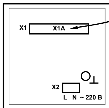
Рисунок Б.1 – Подключение клеммно-блочного соединителя КБ3-25-11-0,75 к индикатору ИТМ-22У (ИТМ-20У)
