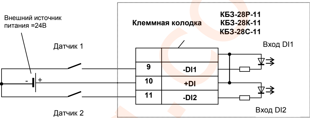
Рисунок Б.21 – Подключение дискретных входов (датчиков) к индикатору с помощью КБ3-28P-11, КБ3-28K-11 или КБ3-28C-11
