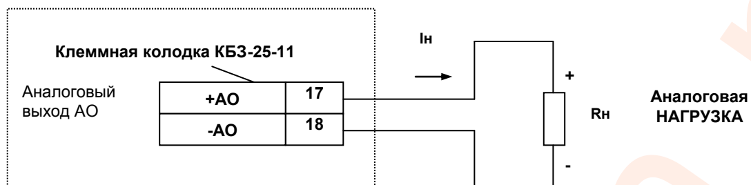
Рисунок Б.10 – Подключение аналоговых нагрузок с помощью КБ3-25-11
