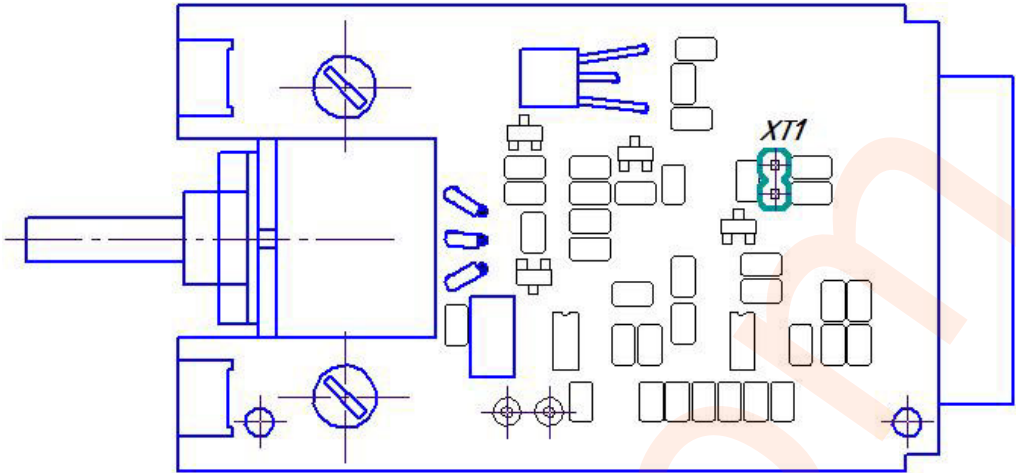
Рисунок 3. Размещение перемычек выбора входных сигналов и контрольных точек
