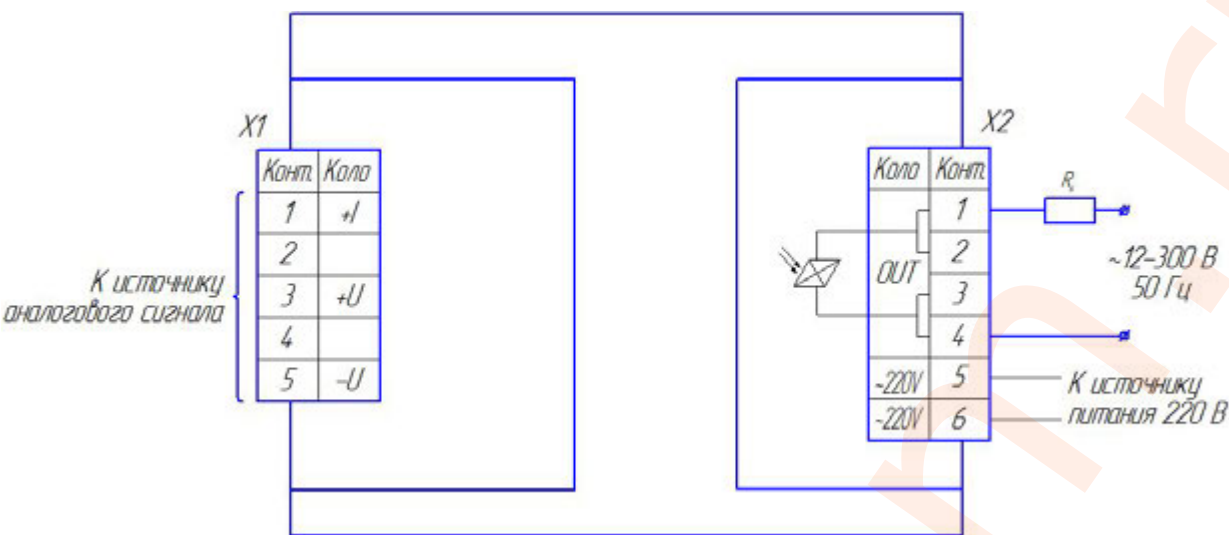
б) Рисунок 4. Схема электрических подключений температурного регулятора МИК-1-200: а) для релейного исполнения регулятора; б) для оптосимисторного исполнения регулятора.
