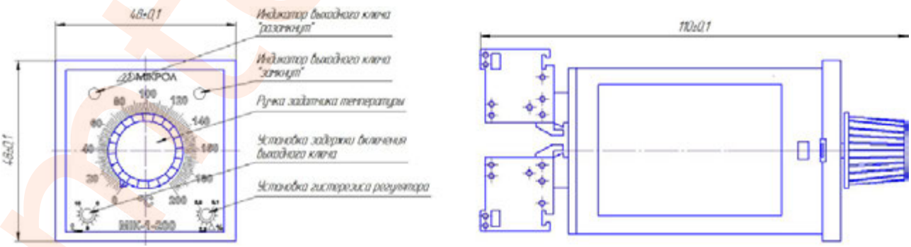
Рисунок 1- Температурный регулятор МИК-1-200 Внешний вид
