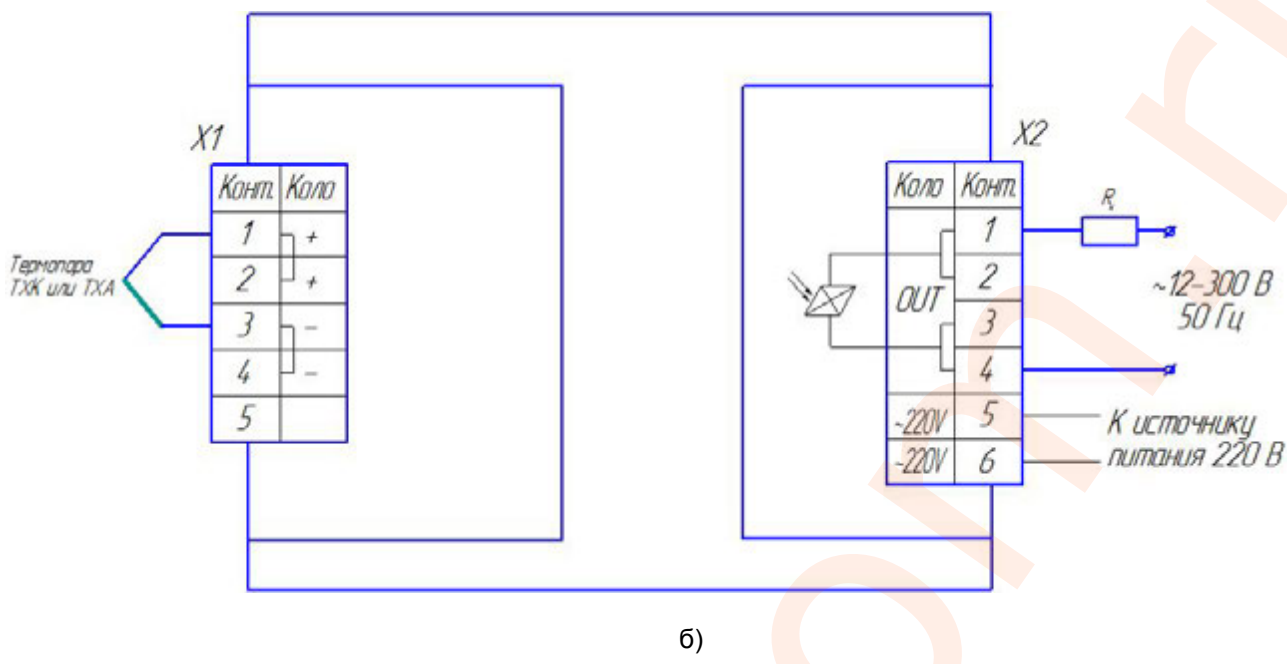
Рисунок 4. Схема электрических подключений температурного регулятора МИК-1-400: а) для релейного исполнения регулятора; б) для оптосимисторного исполнения регулятора.
