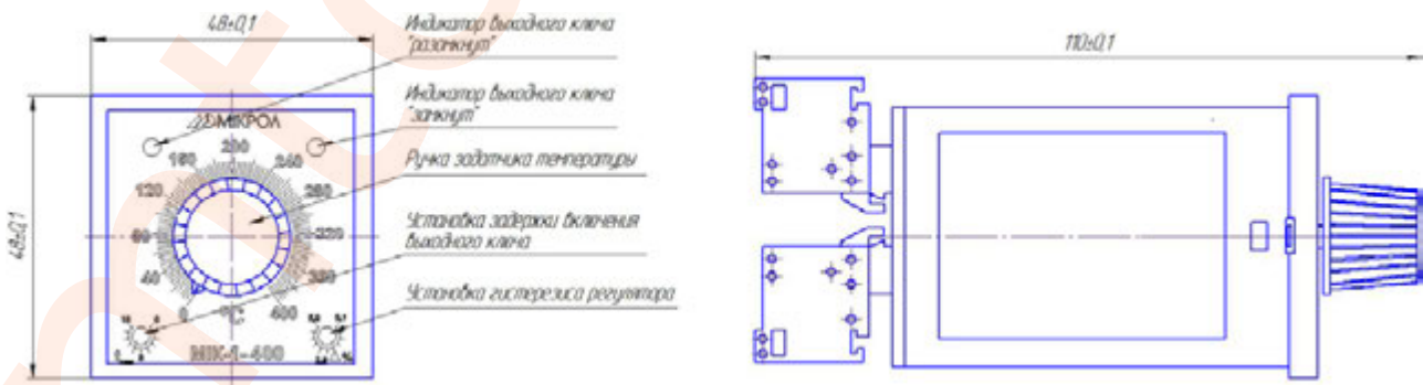
Рисунок 1- Температурный регулятор МИК-1-400 Внешний вид
