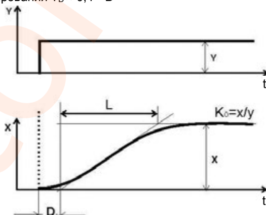
Рисунок 4.8 - Переходная функция объекта регулирования с самовывравниванием
