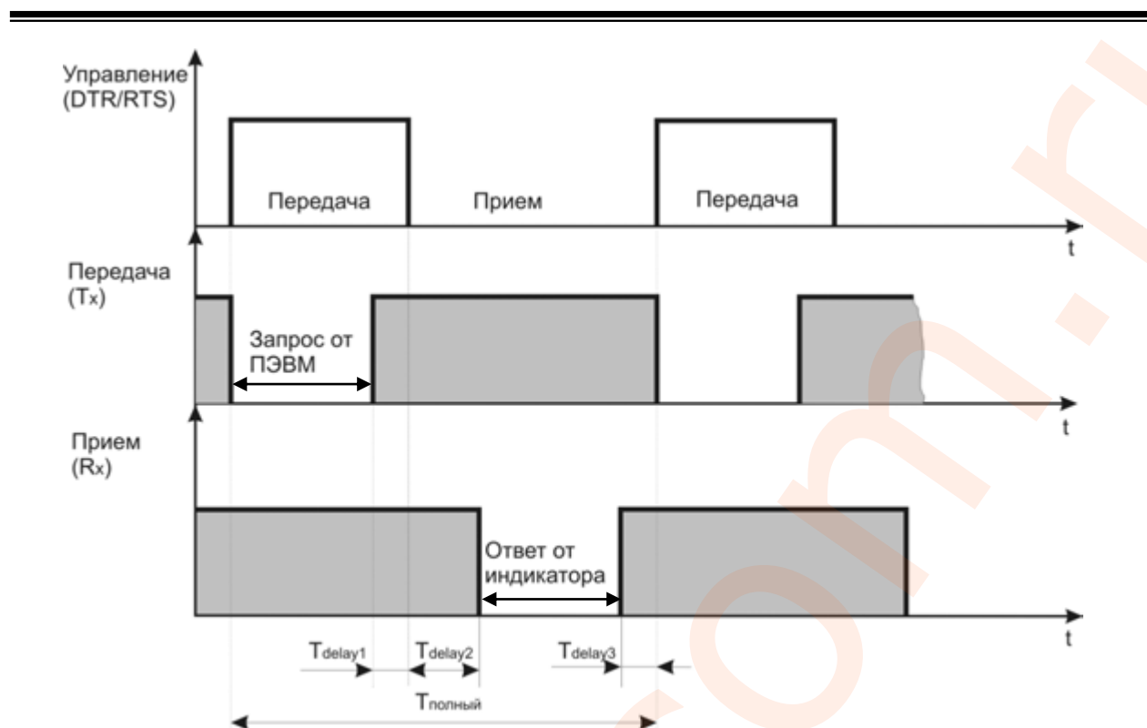
Рисунок В.1 - Временные диаграммы управления передачей и приемом блока интерфейсов БПИ-485 (БПИ-52)
