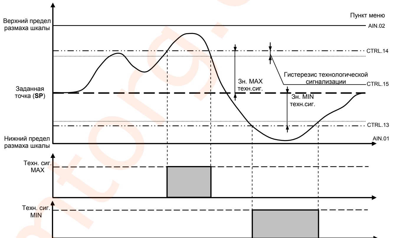
Рисунок 3.12 - График срабатывания девиационной технологической сигнализации п. CTRL.12=0001
