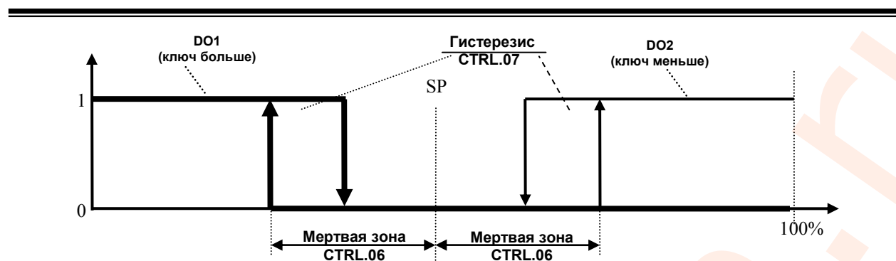
Рисунок 3.9 - График работы дискретных выходов 3-х позиционного регулятора с использованием зоны нечувствительности (CTRL.06)
