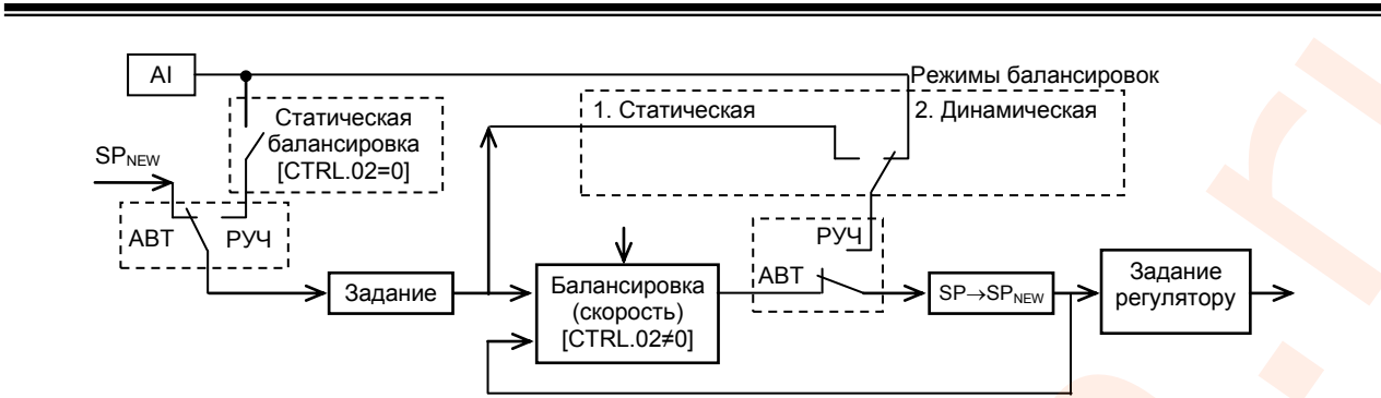
Рисунок 4.2 - Функциональная схема балансировок регулятора МИК-111
