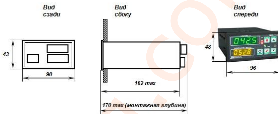
Рисунок А.2 - Габаритные размеры регулятора МИК-112
