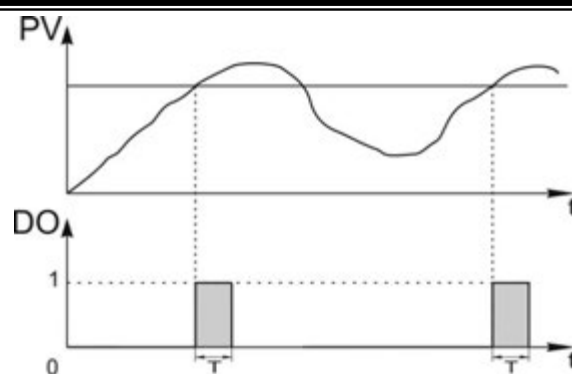
Рисунок 3.17 – График работы дискретного выхода при импульсном типе выходного сигнала
