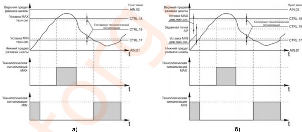
Рисунок 3.18 - График срабатывания:
