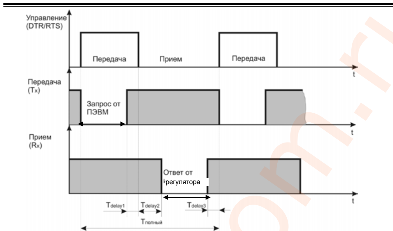
Рисунок В.1 - Временные диаграммы управления передачей и приемом блока интерфейсов БПИ-485 (БПИ-52)
