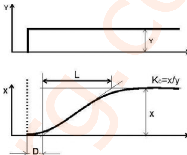
Рисунок 4.8 - Переходная функция объекта регулирования с самовыравниванием
