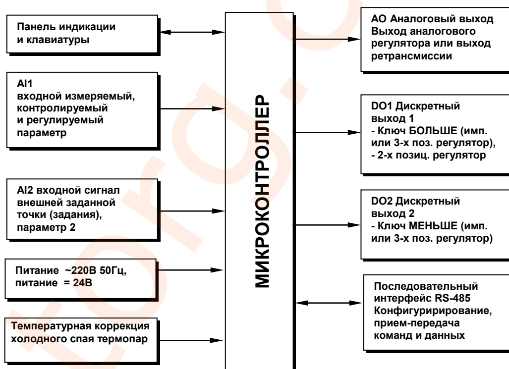
Рисунок 3.2 – Структурная схема регулятора МИК-112
