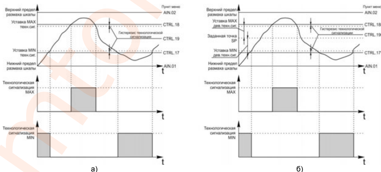
Рисунок 3.20 - График срабатывания:
