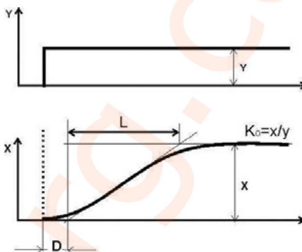
Рисунок 4.7 - Переходная функция объекта регулирования с самовыравниванием
