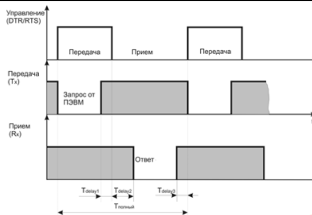
Рисунок В.1 - Временные диаграммы управления передачей и приемом блока интерфейсов БПИ-485 (БПИ-52)
