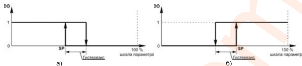
Рисунок 3.16 – Пример работы выходного устройства: а) по логике обратного 2-х позиционного управления п. CTRL.00=0000, п. CTRL.01=0000, б) по логике прямого 2-х позиционного управления п. CTRL.00=0000, п. CTRL.01=0001
