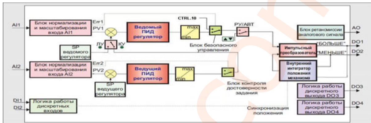
Рисунок 3.12 – Структурная схема каскадного импульсного регулятора
