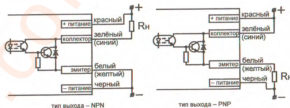
Рис.2. Схемы подключения фотодатчика МикРА Ф2Б.
