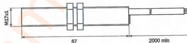
Рис.1. Габаритные размеры излучателя МикРА Ф4И и приемника МикРА Ф4П
