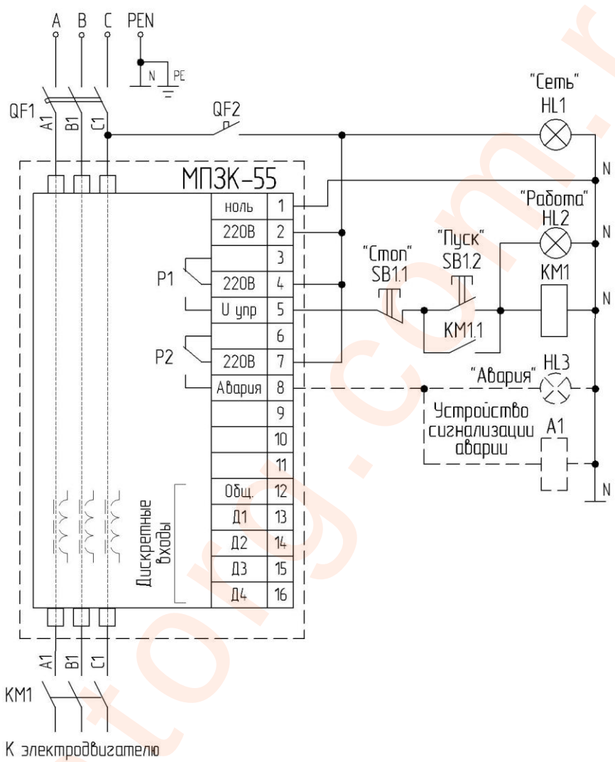
Рис.2 Схема подключения МПЗК-55
