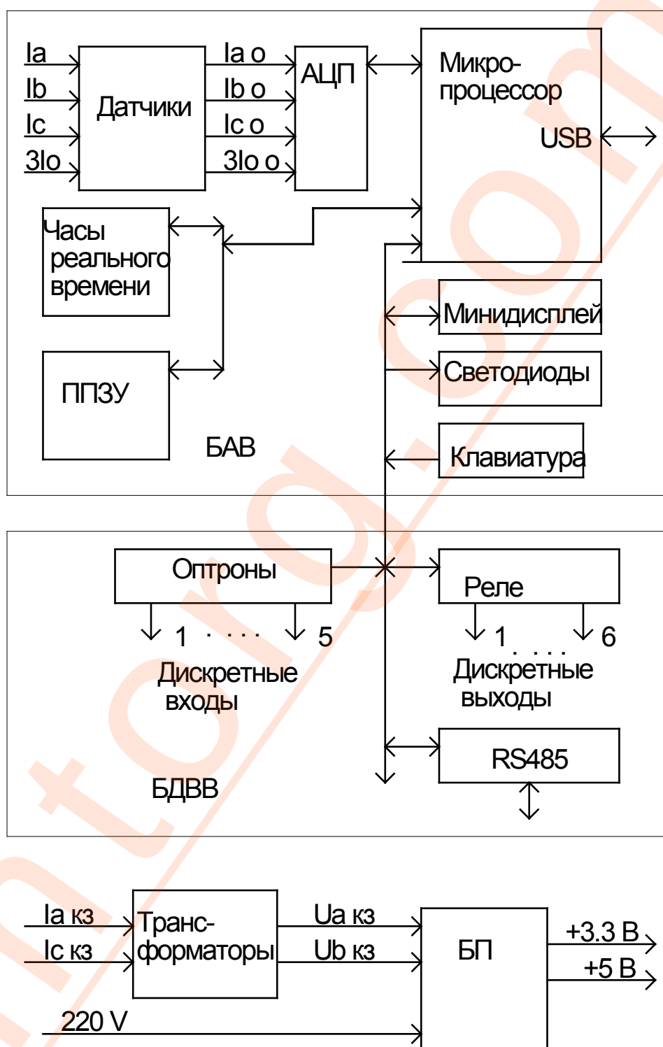
Рис. 11 Структурная схема МРЗС-05Л
