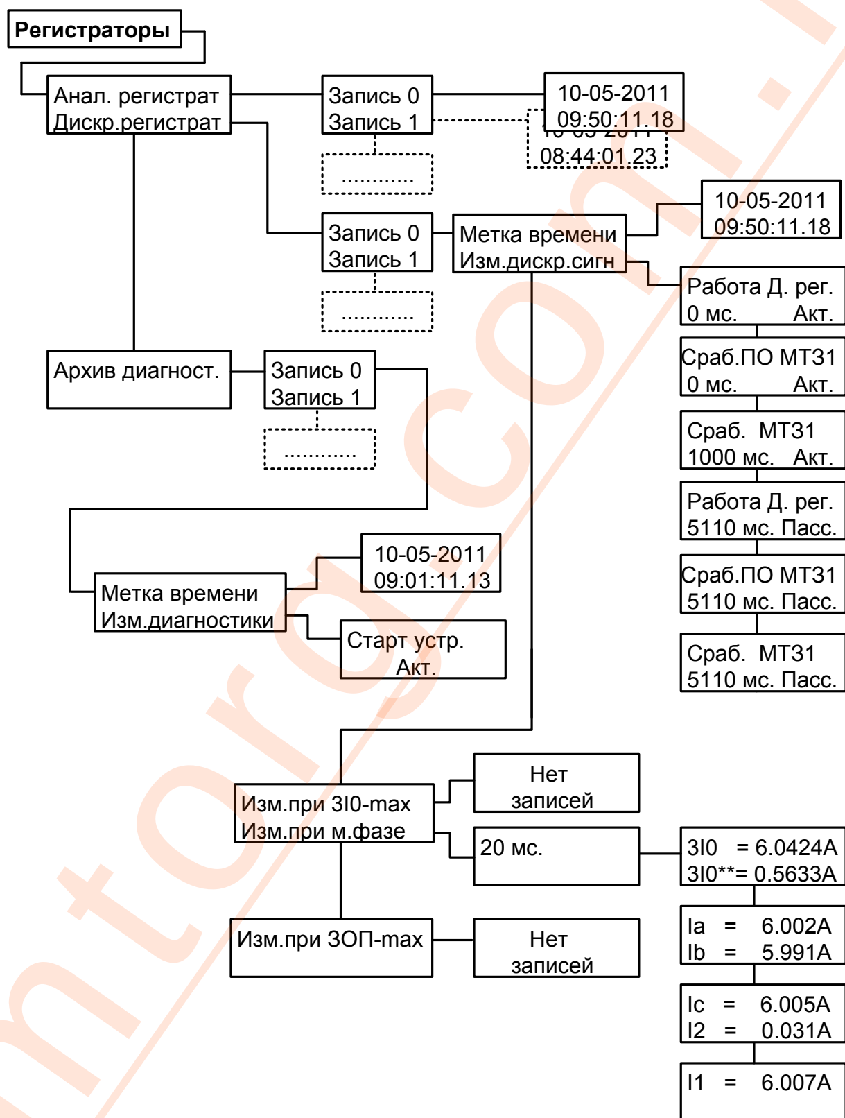
Рис. 25 Структура пункта меню «Регистраторы»
