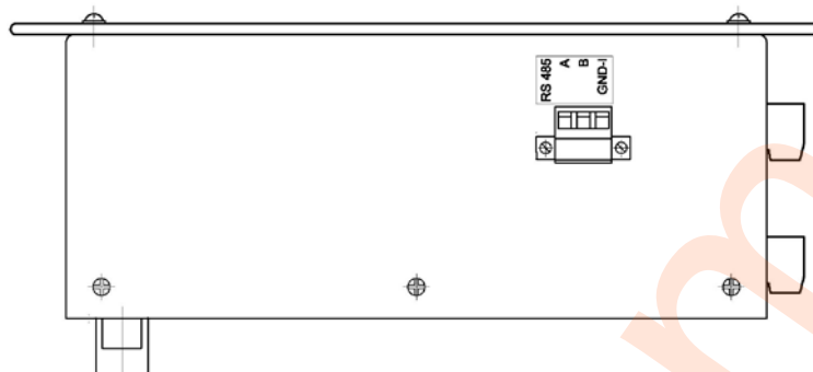
Рис.7 Вид снизу МРЗС-05Л АИАР.466452.001
