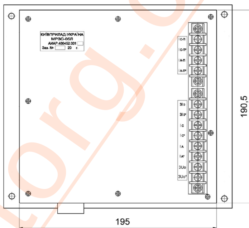
Рис.8 Вид сзади МРЗС-05Л АИАР.466452.001
