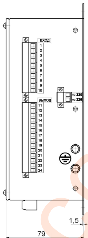
Рис.3 Вид справа МРЗС-05Л АИАР.466452.001-01
