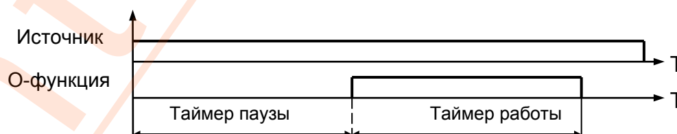
Рис. 19 Диаграмма работы определяемой функции, тип функции – прямая
