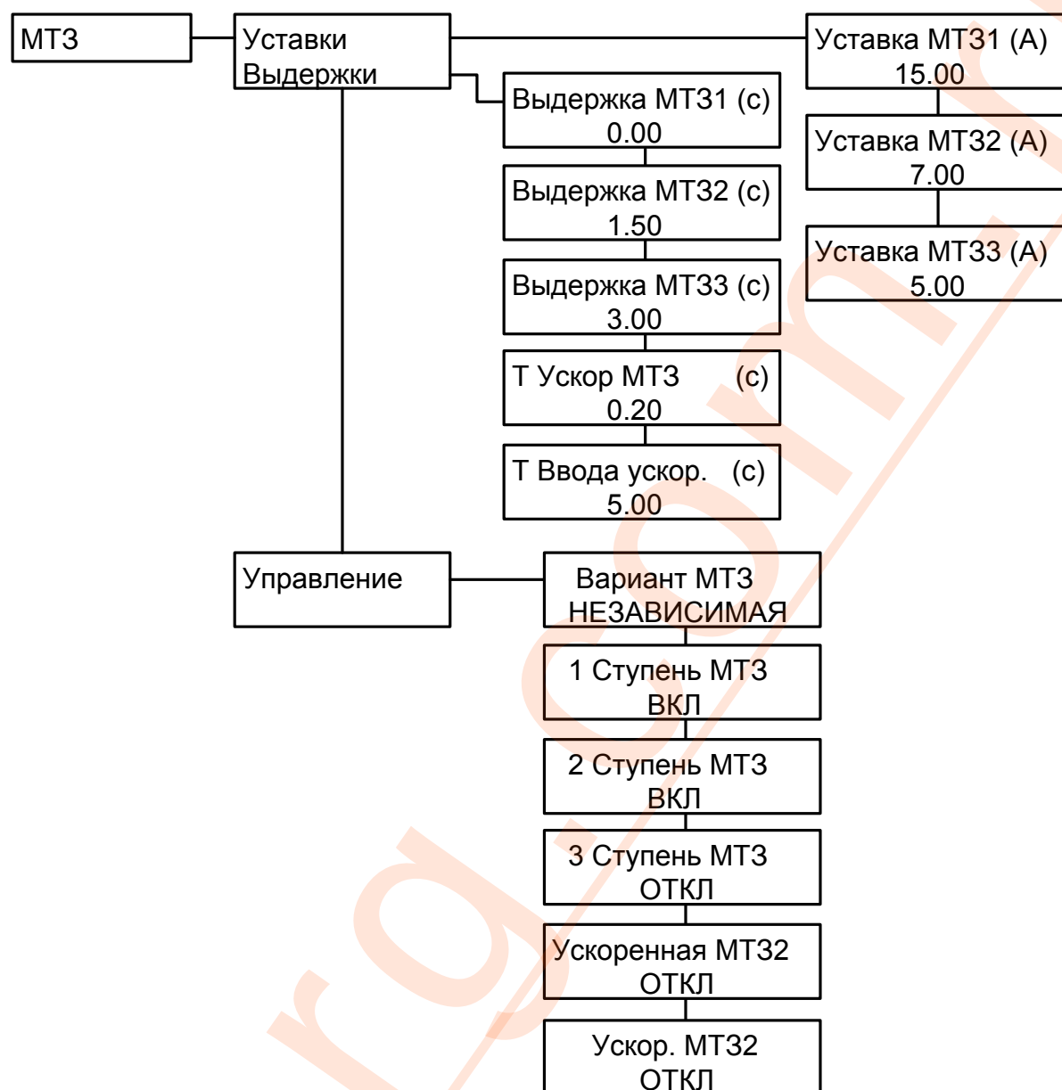
Рис. 31 Структура пункта меню «МТЗ»
