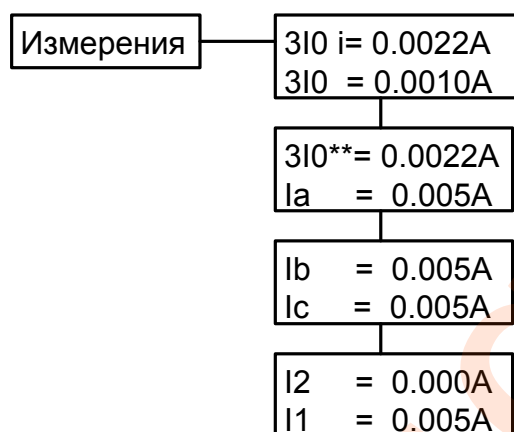
Рис. 23 Структура пункта меню «Измерения»
