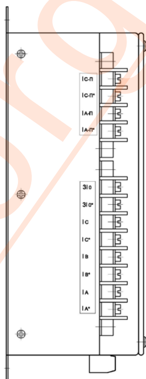
Рис. 2 Вид слева МРЗС-05Л АИАР.466452.001-01
