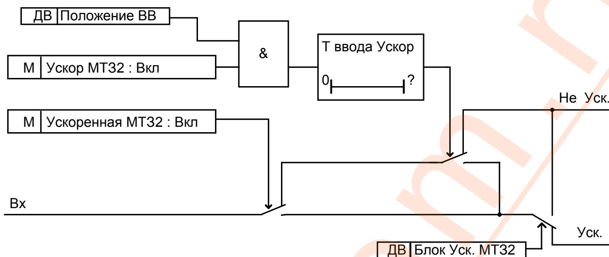
Рис. 13 Функциональная схема блока ускорения МТЗ
