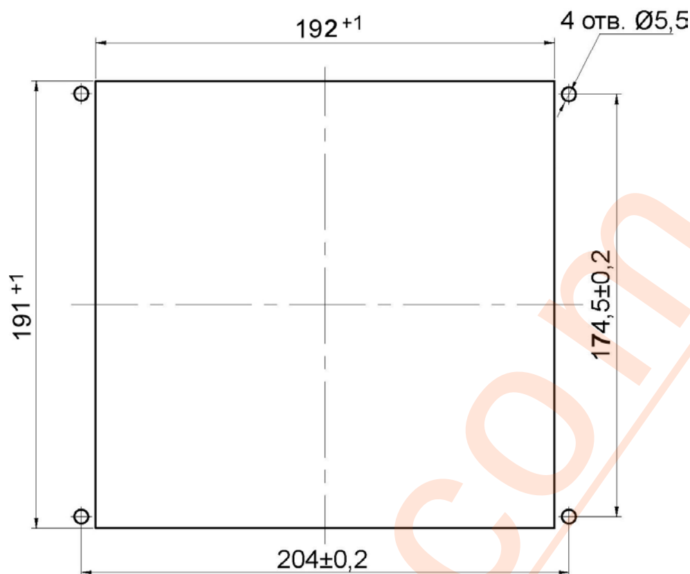
Рис.9 Разметка панели под установку устройства МРЗС-05Л АИАР.466452.001
