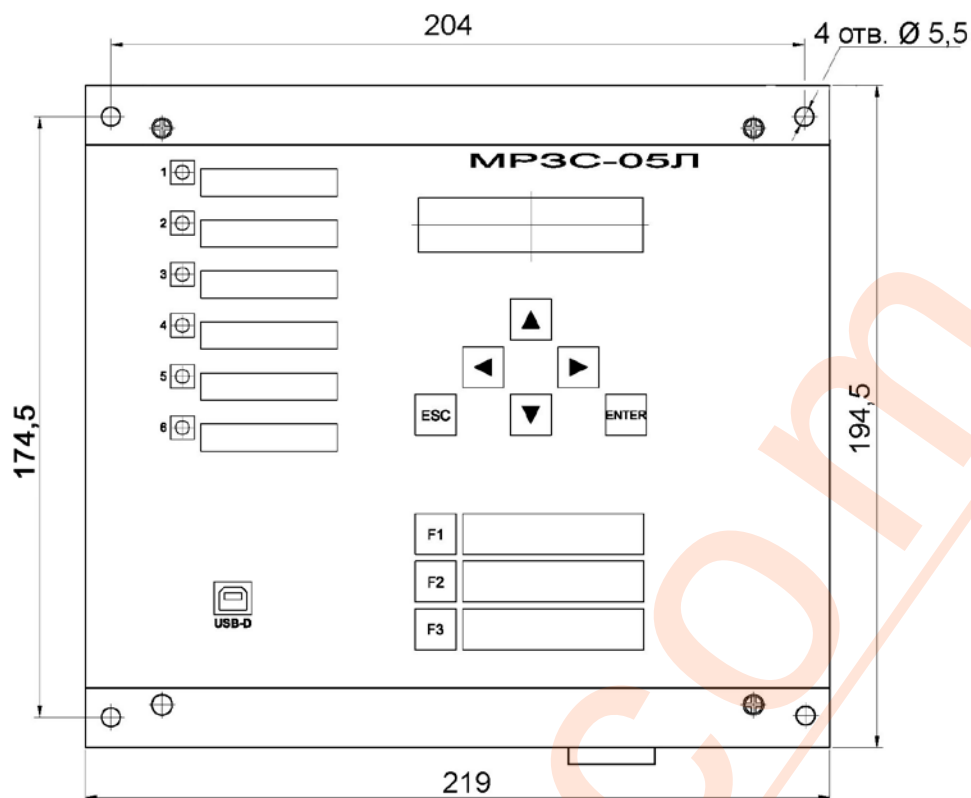
Рис.5 Вид спереди МРЗС-05Л АИАР.466452.001
