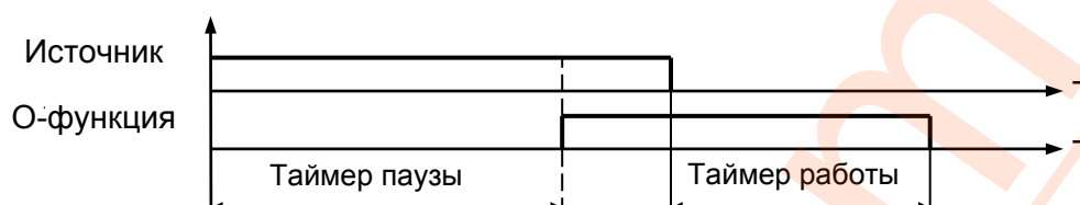
Рис. 20 Диаграмма работы определяемой функции, тип функции - обратная
