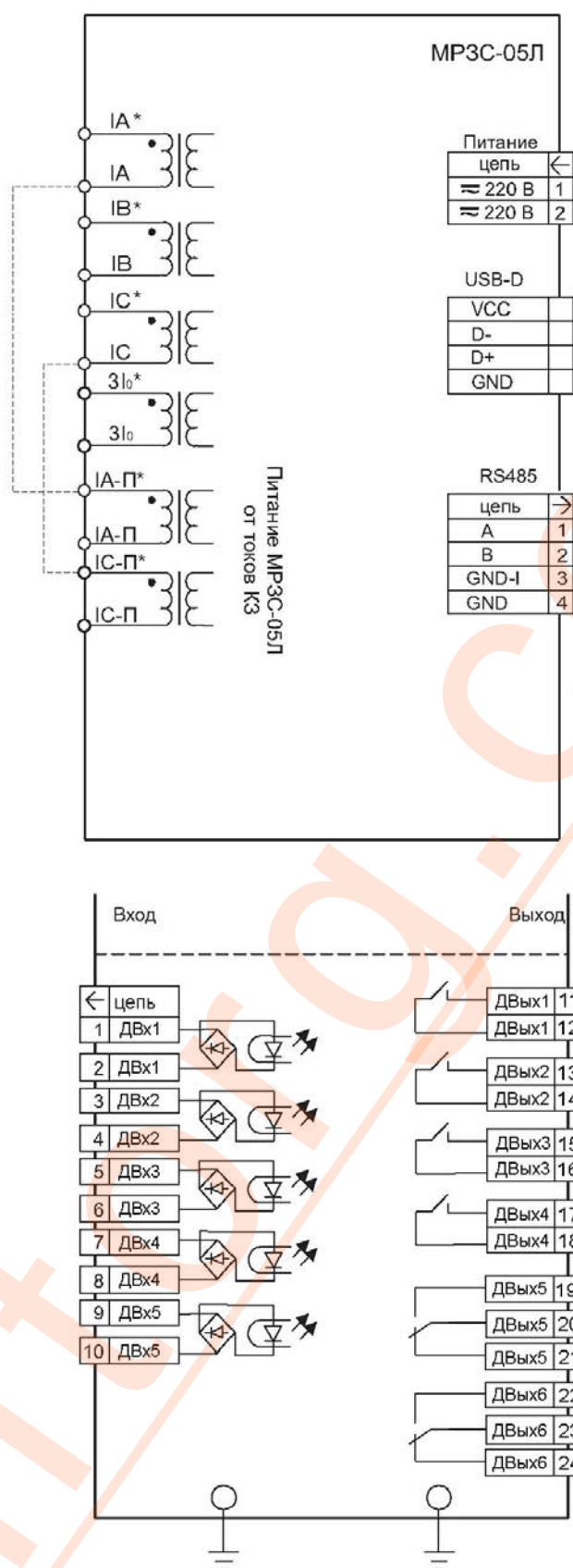
Рис. 10 Упрощенная схема подключения МРЗС-05Л
