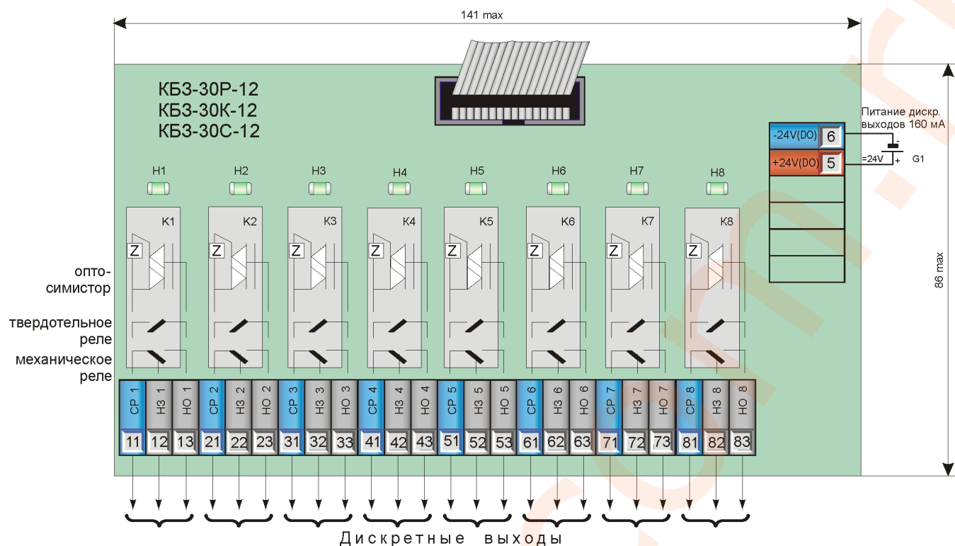
Рисунок Б.3.11 - Подключение сигналов модуля расширения МР-51-03 с помощью клеммно-блочного соединителя КБ3-30P-12, КБ3-30K-12, КБ3-30C-12
