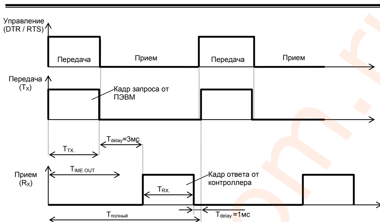
Рисунок 7.1. Временные диаграммы управления передачей и приемом блока интерфейсов БПИ-485.
