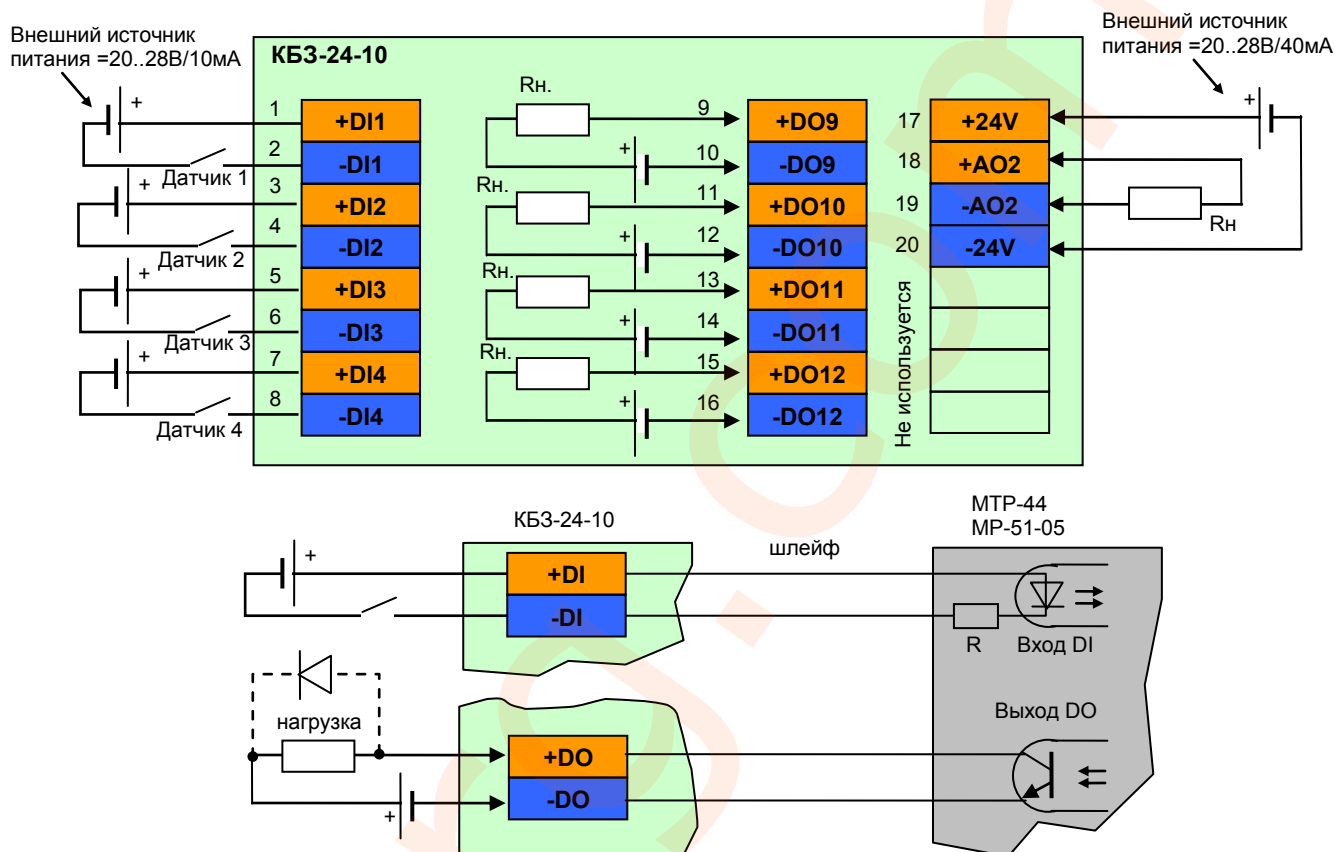
Рисунок Б.3.13 - Подключение сигналов модуля расширения MP-51-05 с помощью клеммно-блочного соединителя KB3-24-10
