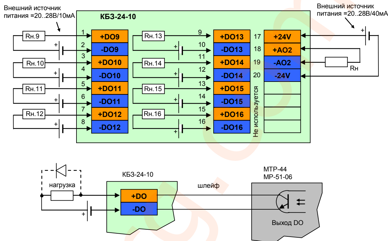
Рисунок Б.3.15 - Подключение сигналов модуля расширения МР-51-06 с помощью клеммно-блочного соединителя KB3-24-10
