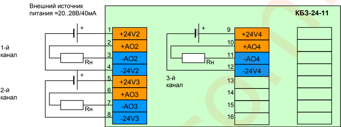
Рисунок Б.3.2.10 - Подключение сигналов модуля расширения МР-51-07 с помощью клеммно-блочного соединителя КБ3-24-11
