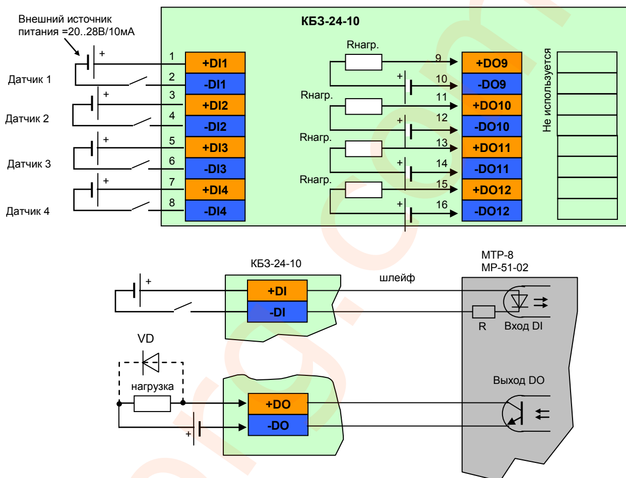
Рисунок Б.3.2.2 - Подключение сигналов модуля расширения МР-51-02 с помощью клеммно-блочного соединителя KB3-24-10
