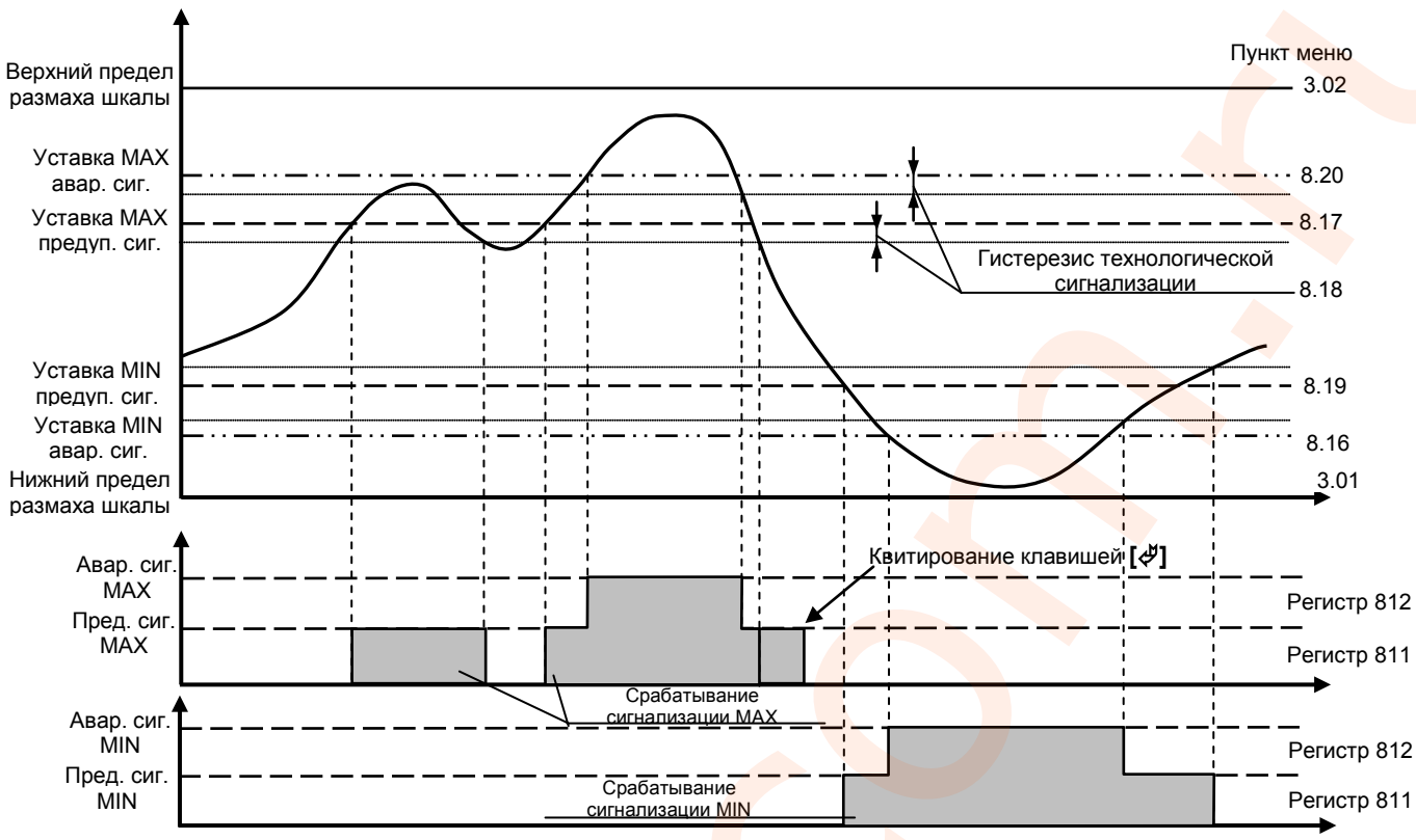
Рисунок 5.11 - График срабатывания абсолютной сигнализации с запоминанием или без п.8.15=0000, 0002
