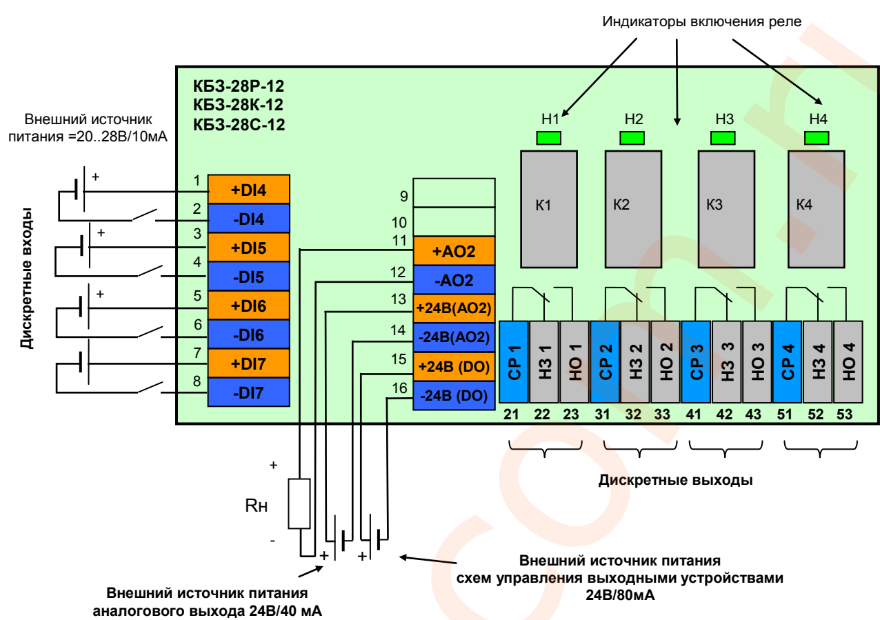
Рисунок Б.3.2.7 - Подключение сигналов модуля расширения МР-51-05 с помощью клеммно-блочного соединителя КБ3-28Р-12, КБ3-28С-12, КБ3-28К-12
