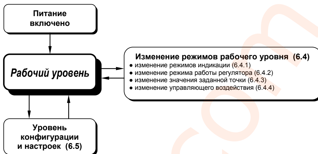
Рисунок 6.1 - Диаграмма уровней работы, защиты и настроек регулятора МТР-8
