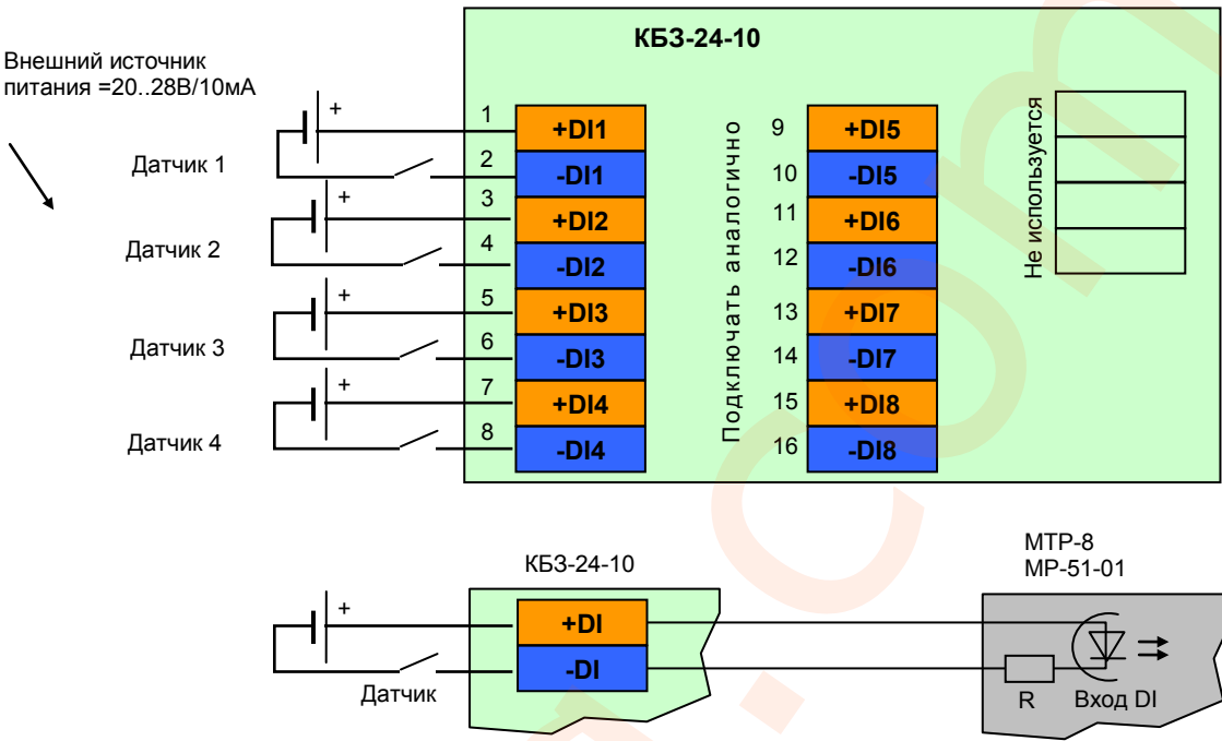
Рисунок Б.3.2.1 - Подключение сигналов модуля расширения МР-51-01 с помощью клеммно-блочного соединителя KB3-24-10
