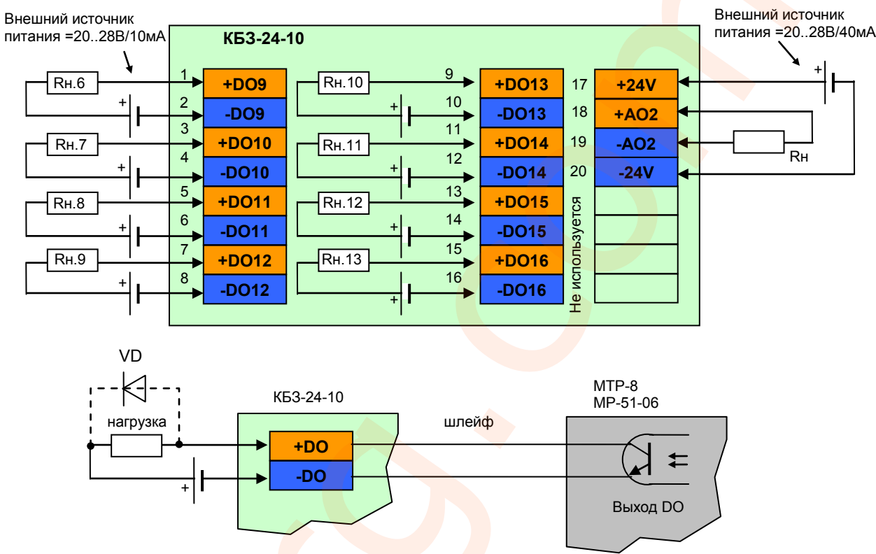
Рисунок Б.3.2.8 - Подключение сигналов модуля расширения МР-51-06 с помощью клеммно-блочного соединителя КБ3-24-10
