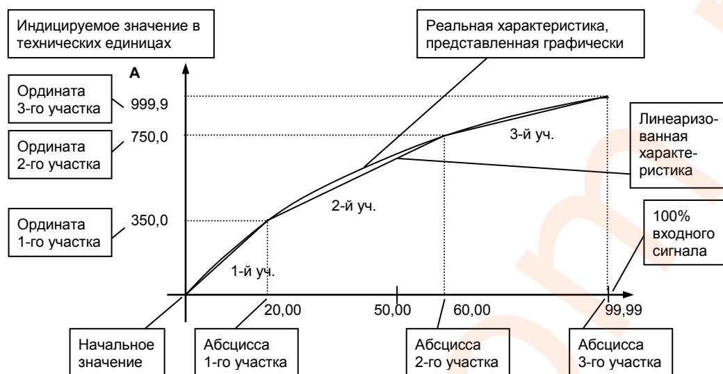
Рисунок 5.3.1 - Линейаризация сигнала, подаваемого на функциональный блок нормализации и масштабирования, представленная графически (кривой)
