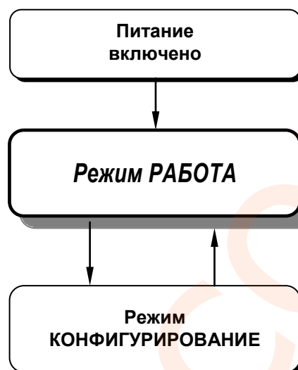
Рисунок 4.6.1 – Диаграмма режимов работы и настройки преобразователя ПНС-13
