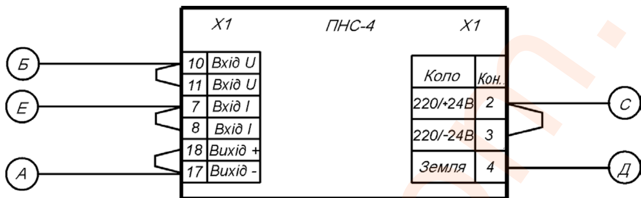
Рисунок 1.1. Схема проверки сопротивления изоляции ПНС-4
