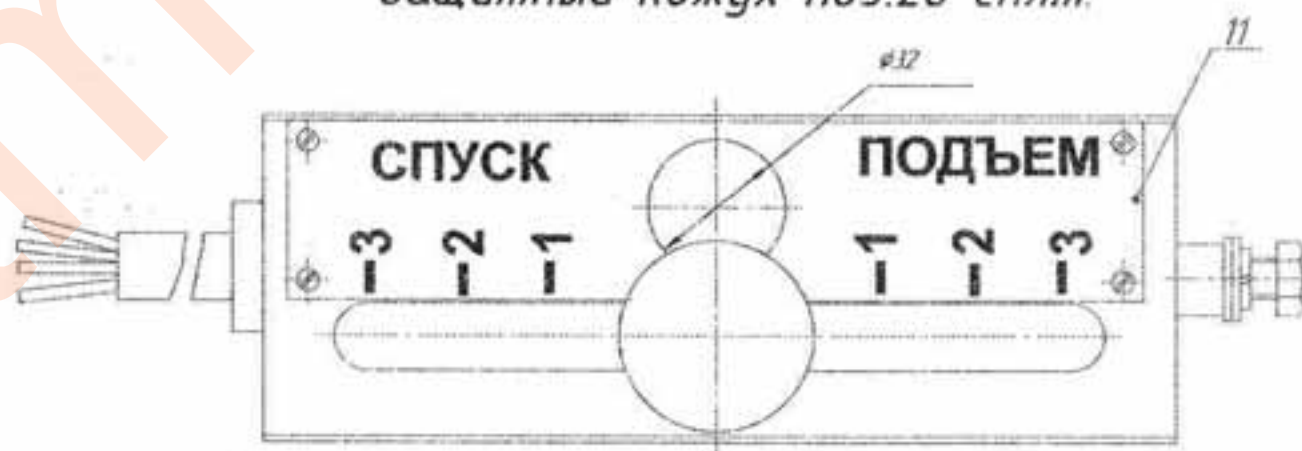
Рисунок 1 - Общий вид командопарата КАГВ-2 (44.67173-2ТТ).
