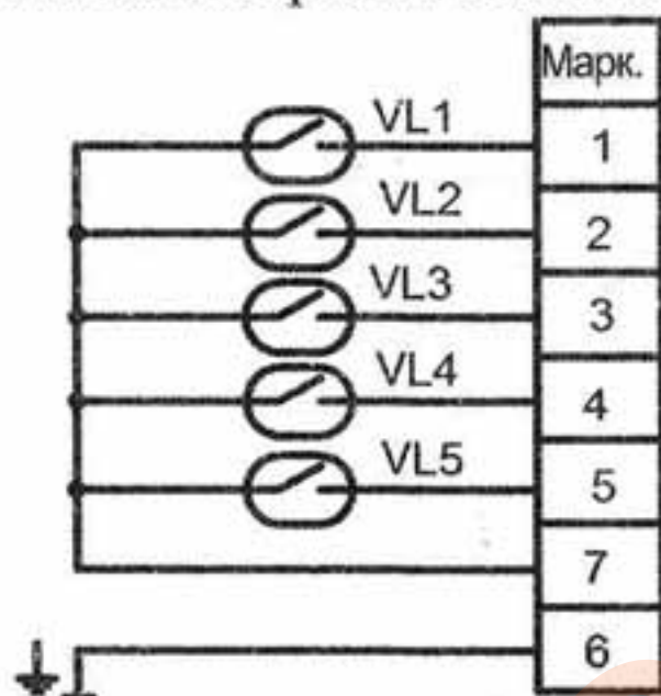
Рисунок 3 – Схема электрическая принципиальная командоаппарата (44.67173-2ТТ)
