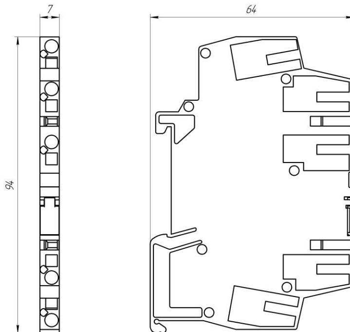
Рисунок 1.1 – Внешний вид и габаритные размеры преобразователя ППМ-645
