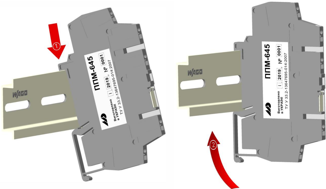
Рисунок 3.2 – Схема крепления преобразователя ППМ-645 на DIN-рейку
