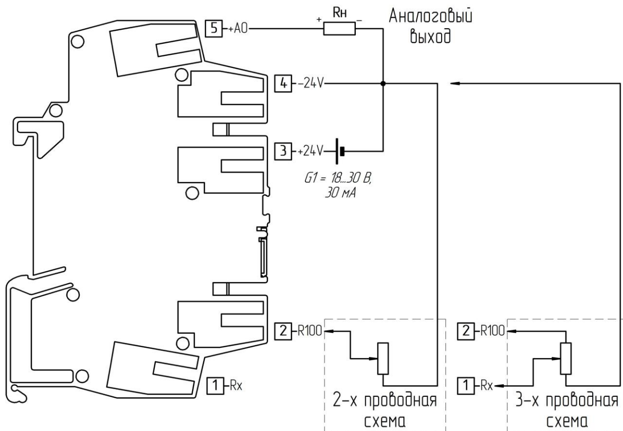
Рисунок 3.4 - Схема внешних соединений преобразователя ППМ-645
