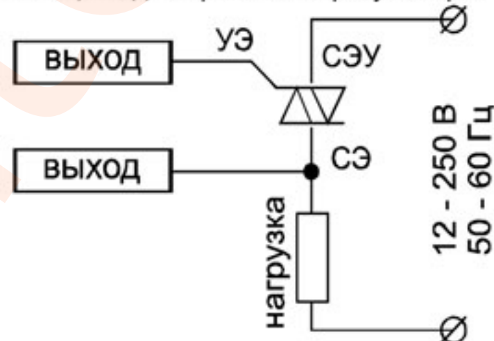
Рис.2. Схема подключения симисторов TC122-25, TC142-80.
