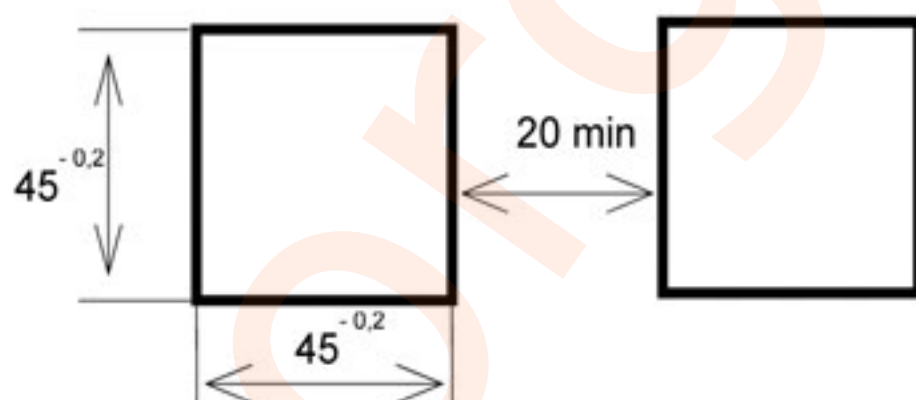
Рис.1. Вырез в щите для крепления регулятора.
