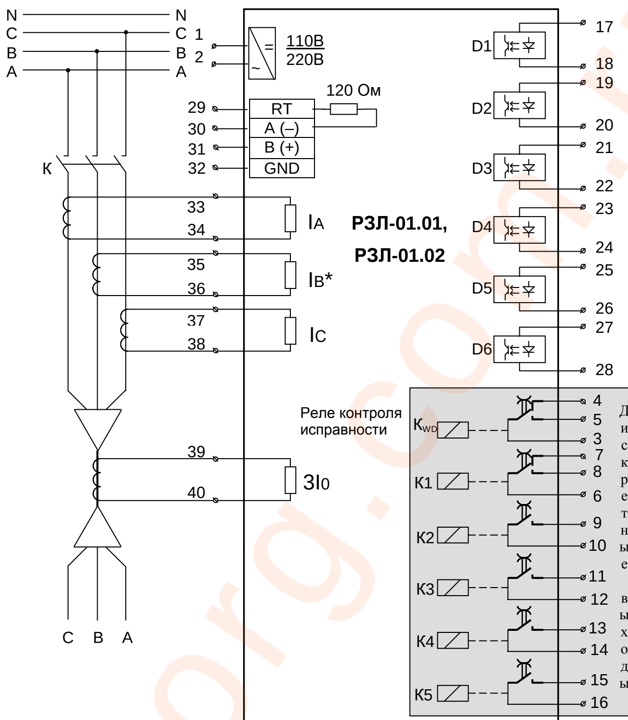
Рисунок 2 Схема подключения внешних цепей к устройству РЗЛ-01.01, РЗЛ-
