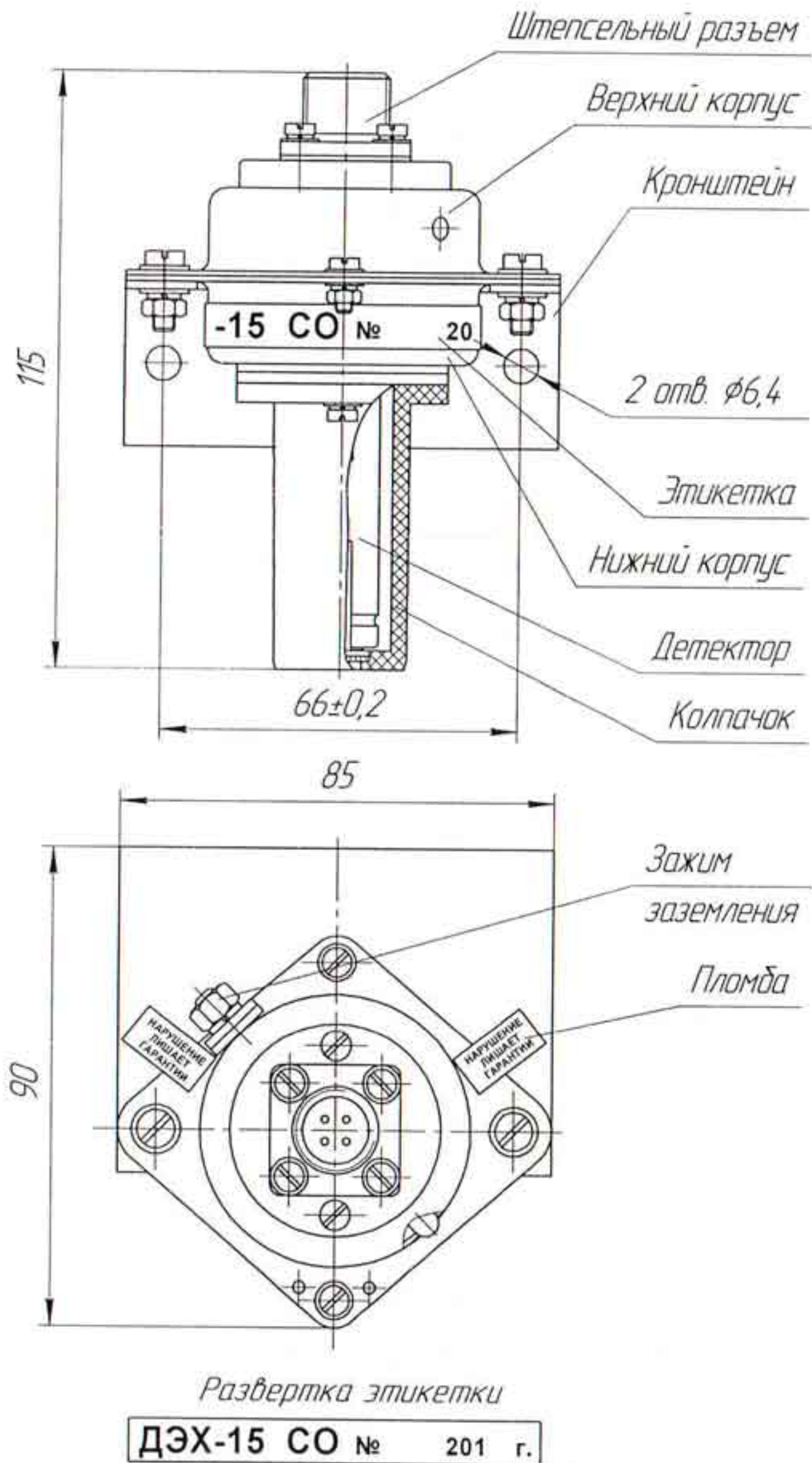
Рисунок А.5 – Общий вид датчика ДЭХ-15
