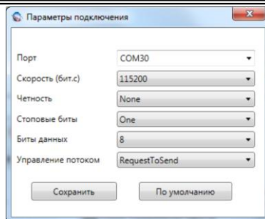
Рисунок 7.3.2 – Окно настроек COM-порта GSM-контроллера Squid-5H-GasWell
