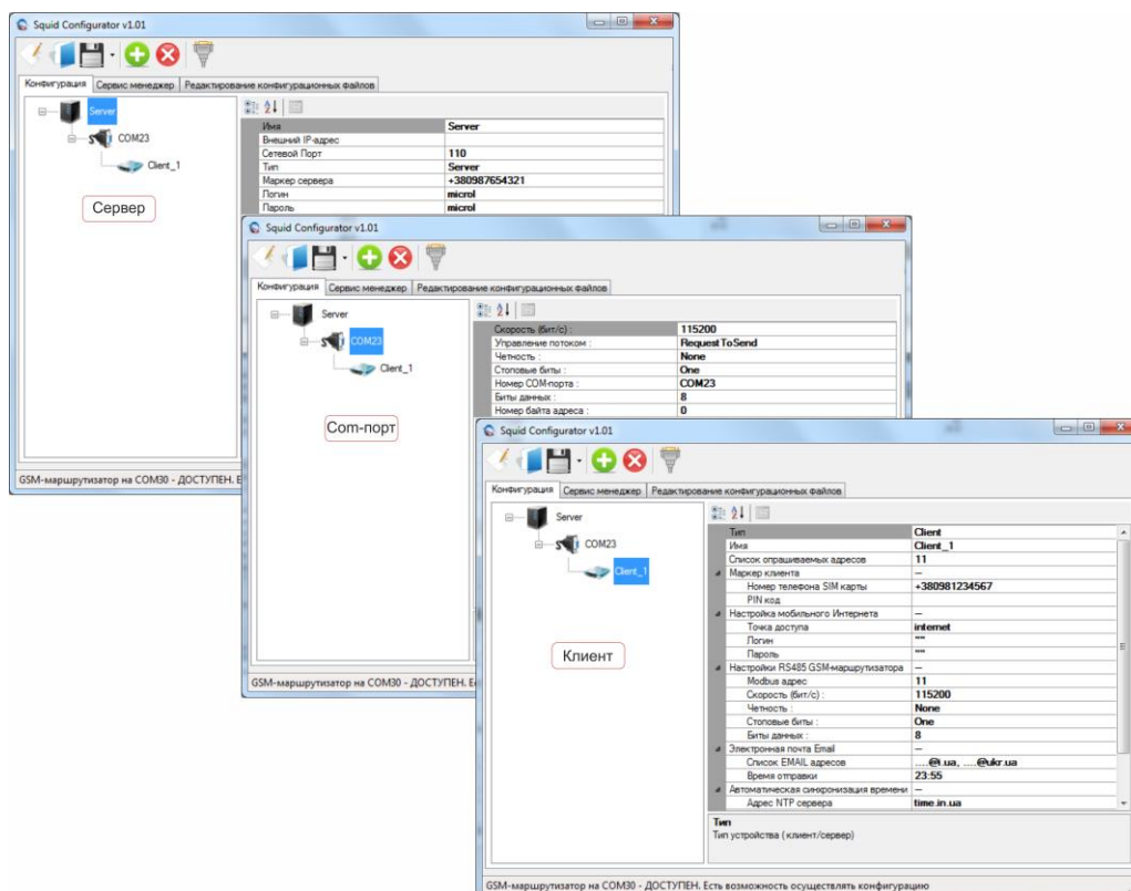
Рисунок 6.2 - Вкладка «Конфигурация»
