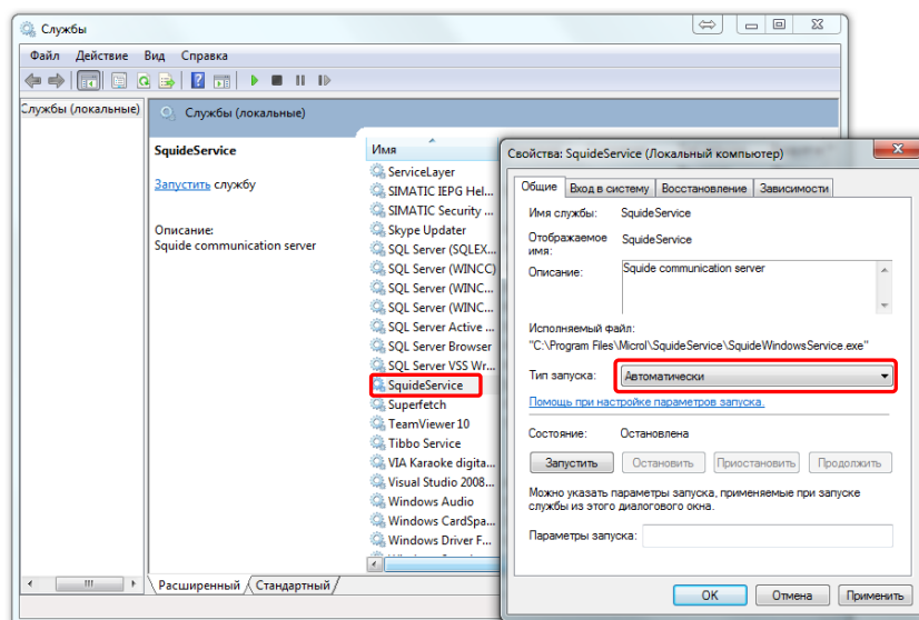
Рисунок 7.5.6 - Включение автоматического запуска сервера
