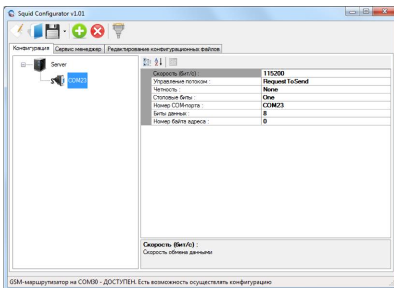
Рисунок 7.2.2 – Добавление виртуального COM порта к серверу
