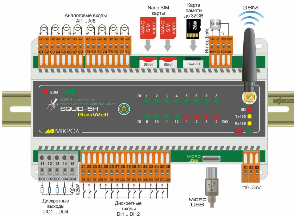
Рисунок А – Схема внешних соединений GSM-контроллера Squid-5H-GasWell
