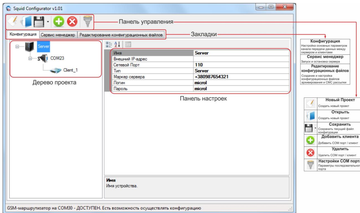
Рисунок 6.1 - Рабочее окно программы Squid-Конфигуратор
