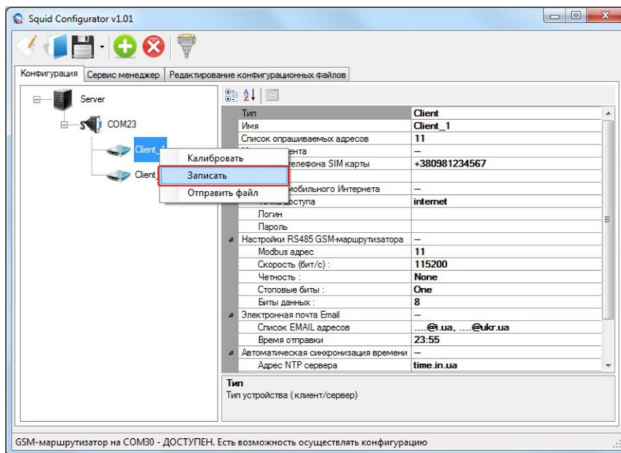
Рисунок 7.3.3 - Запись настроек в GSM-контроллер Squid-5H-GasWell
