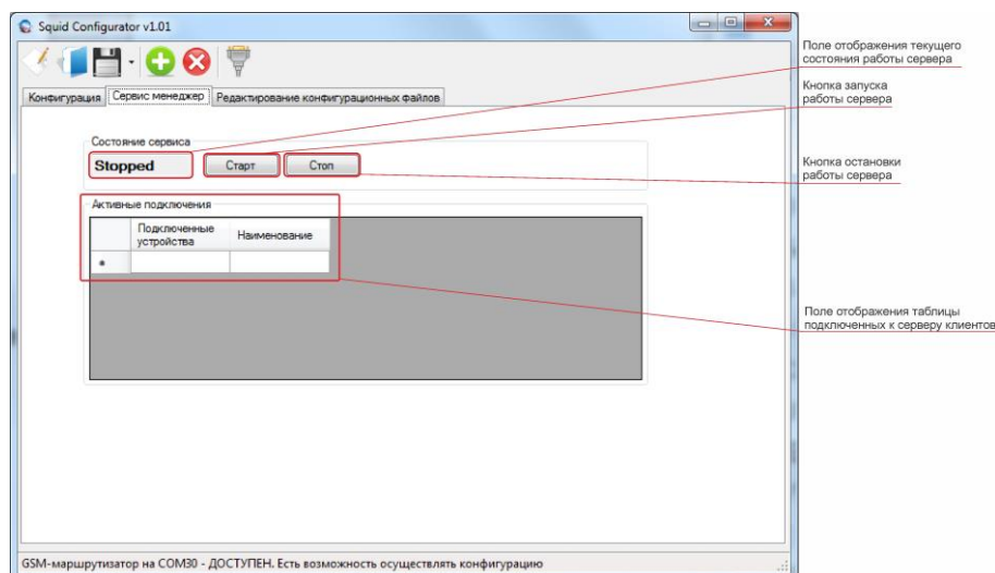
Рисунок 6.3 – Вкладка «Сервис менеджер»
