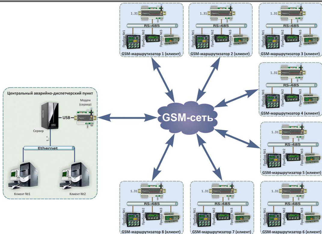
Рисунок 1.2 – Схема системы со Squid-1H в качестве сервера и восемью удаленными GSM-контроллерами Squid-5H-GasWell
