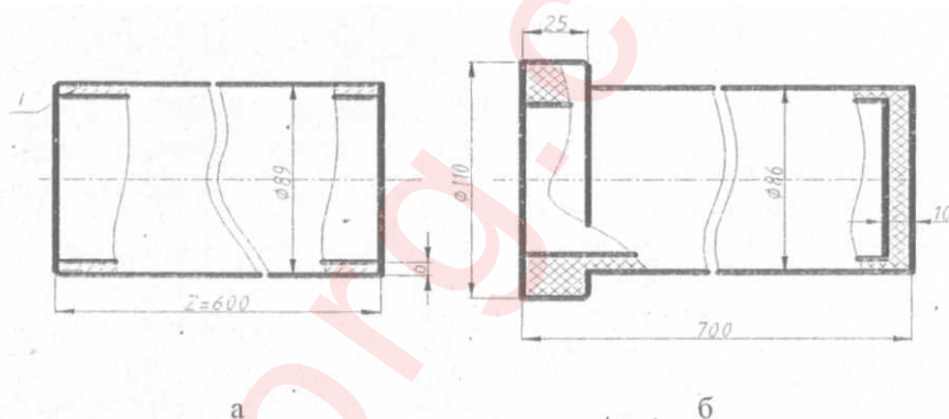
Рис. 3. Труба визирная:
