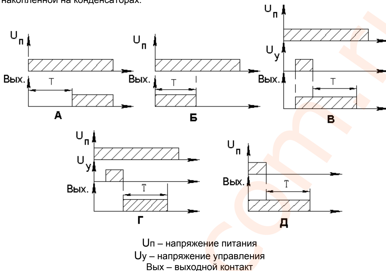
Рисунок 2 – Функциональные диаграммы реле
