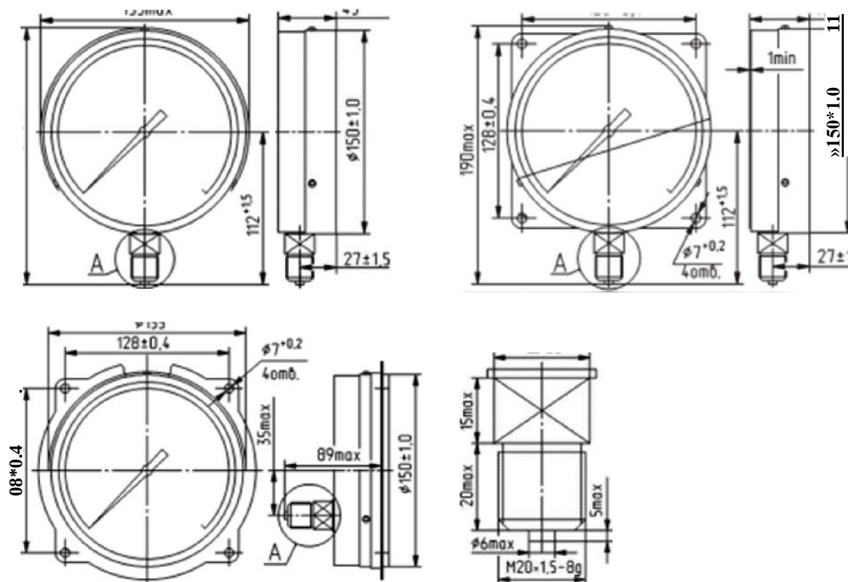
Габаритные и присоединительные размеры МП4А-У2
