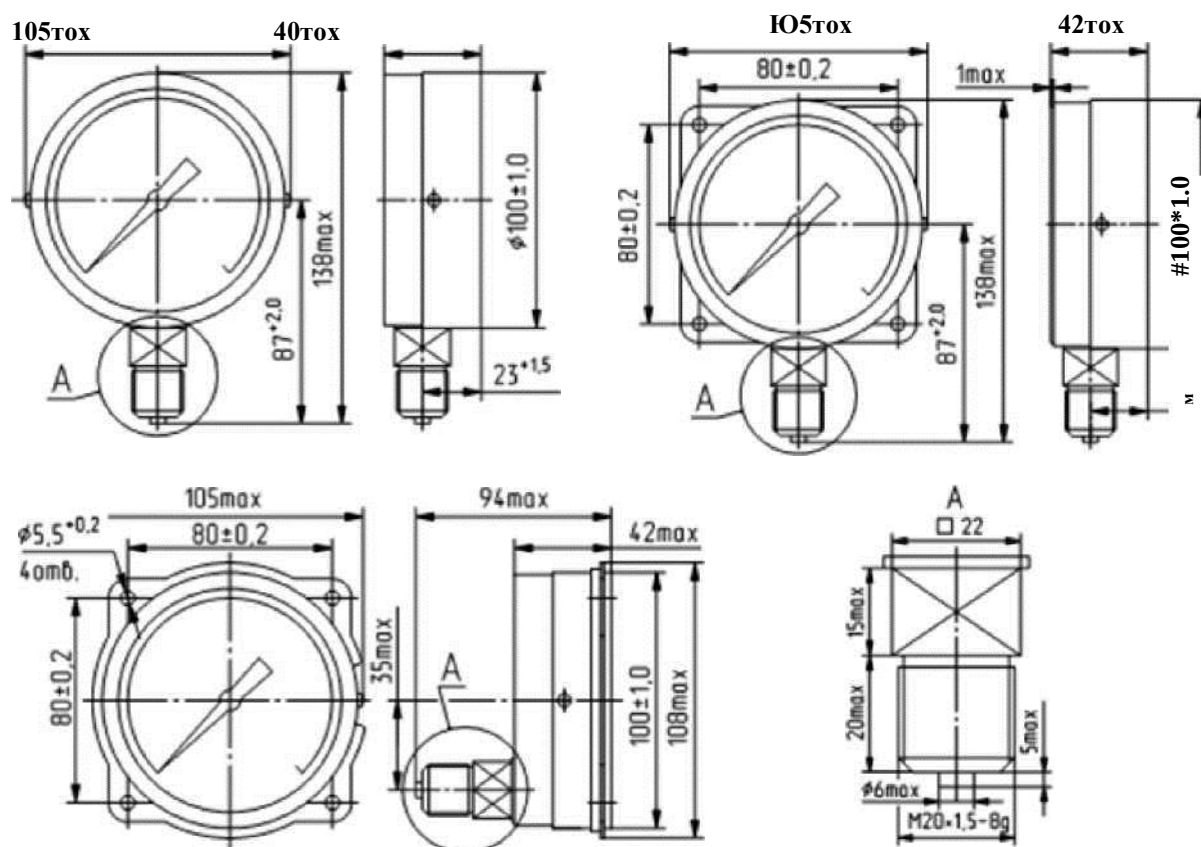
Габаритные и присоединительные размеры МП3А-У2
