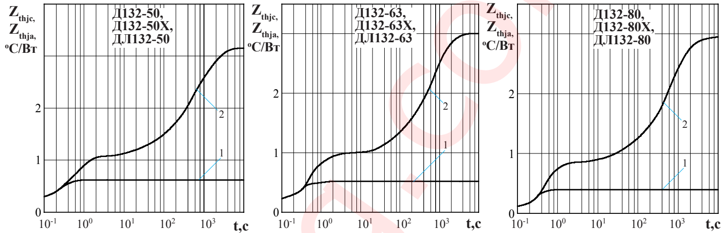
Рисунок 11 - Зависимость теплового сопротивления переход - корпус Z_{thjc} (1) и переход- среда Z_{thja} (2) от времени t при естественном охлаждении T_a = 40 °C на типовом охладителе.
