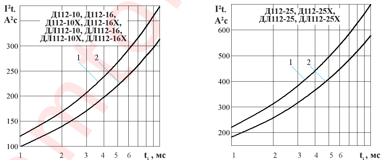
Рисунок 9 - Зависимость защитного показателя \Gamma^2t от длительности импульса тока t_i при исходной температуре структуры T_j = 25 °C (1) и максимальной температуре T_{jm} (2)
