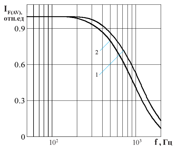
Рисунок 13 - Зависимость допустимого среднего прямого тока I_{F(AV)} от частоты f при естественном охлаждении на типовом охладителе при токе синусоидальной формы с углом проводимости \theta = 180 °эл; \tau_p = 50 мкс (1) при T_j = 150 °C, \tau_p = 60 мкс (2) при T_j = 150 °C.
