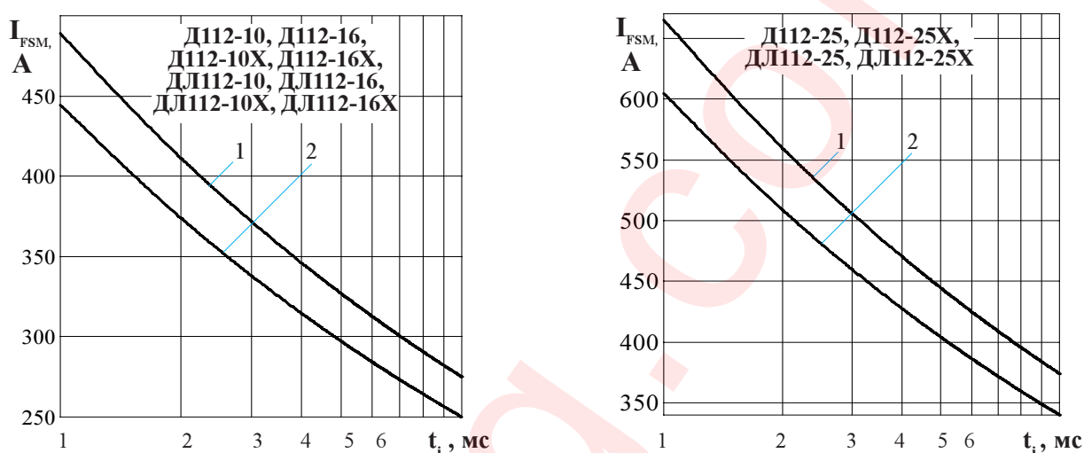
Рисунок 8 - Зависимость допустимой амплитуды ударного прямого тока I_{FSM} от длительности импульса тока t_i при исходной температуре структуры T_j = 25 °C (1) и максимальной температуре T_{jm} (2)
