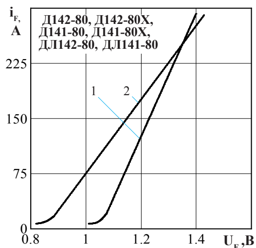
Рисунок 1 - Предельная прямая вольт-амперная характеристика при температуре перехода 25 °C (1) и максимальной температуре перехода T_{жм} (2) I_F = 3,14 I_{F(AV)}
