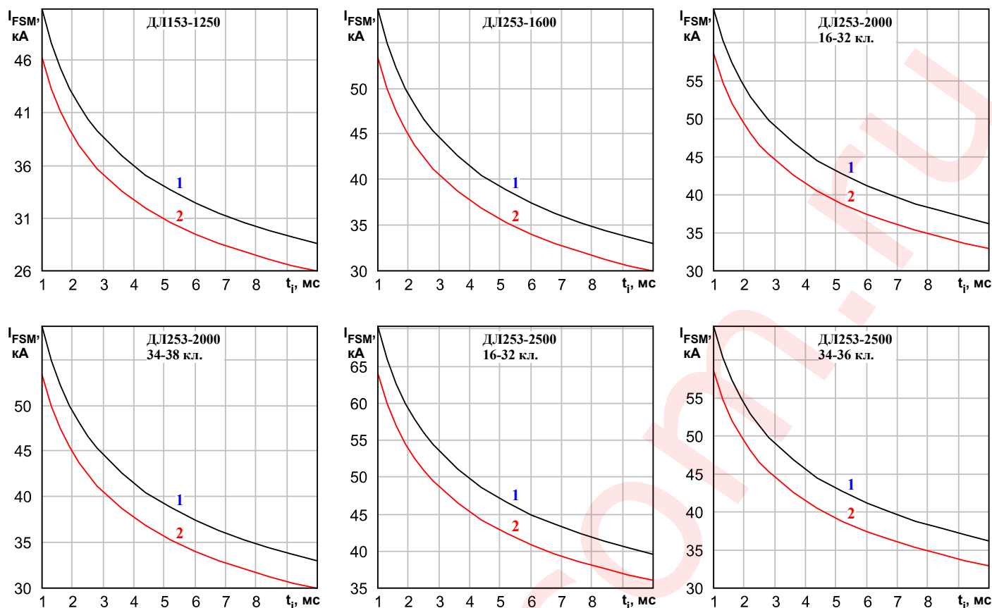
Рисунок 4: Зависимость допустимой амплитуды ударного прямого тока I_{FSM} от длительности импульса тока t_p при исходной температуре структуры T_j = 25^\circ\text{C} (1) и максимально допустимой температуре перехода T_{jm} (2).
