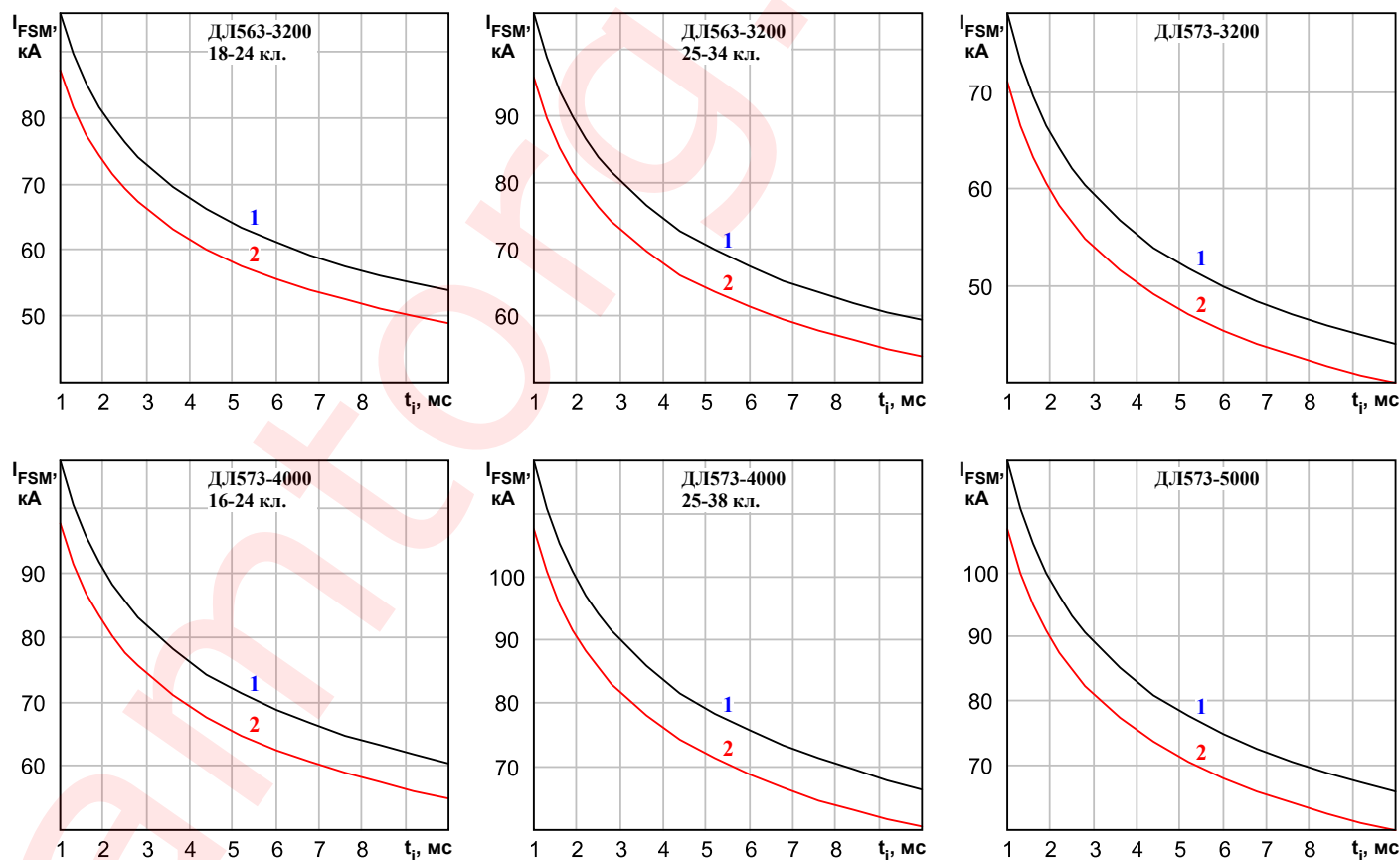
Рисунок 4: Зависимость допустимой амплитуды ударного прямого тока I_{FSM} от длительности импульса тока t_i при исходной температуре структуры T_j = 25^\circ\text{C} (1) и максимально допустимой температуре перехода T_{jm} (2).
