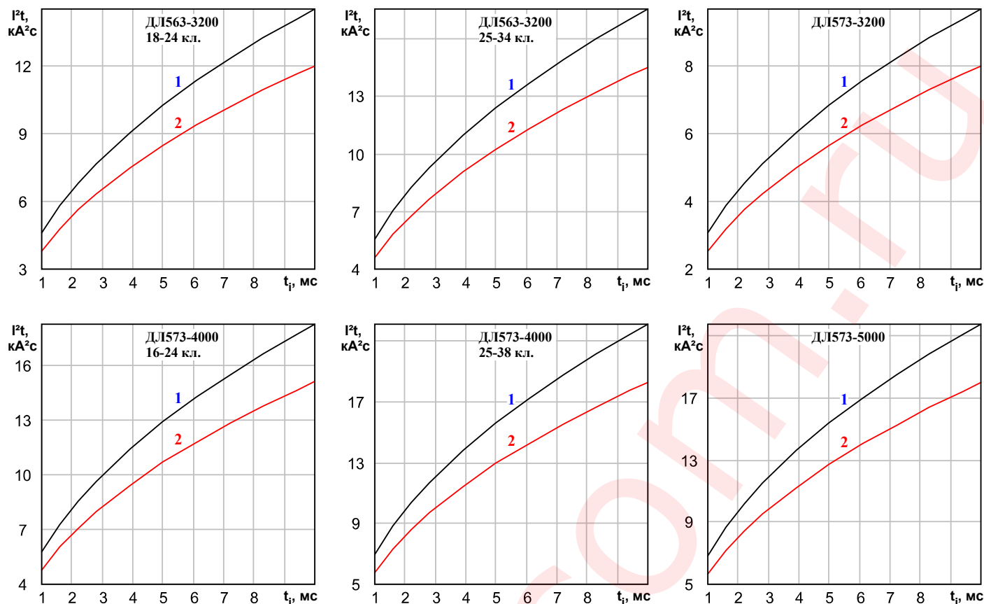
Рисунок 5: Зависимость защитного показателя I^2t от длительности импульса тока t_i при исходной температуре структуры T_j=25^\circ\text{C} (1) и максимально допустимой температуре перехода T_{jm} (2).
