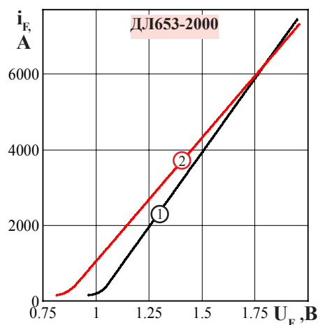
Рисунок 1 - Предельные вольтамперные характеристики при температуре T_j = 25\text{ }^{\circ}\text{C} (1) и максимальной температуре перехода T_{jm} (2)
