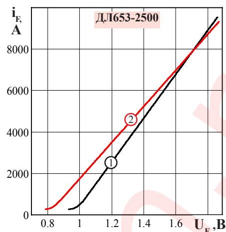
Рисунок 1 - Предельные вольтамперные характеристики при температуре T_j = 25\text{ }^{\circ}\text{C} (1) и максимальной температуре перехода T_{jm} (2)
