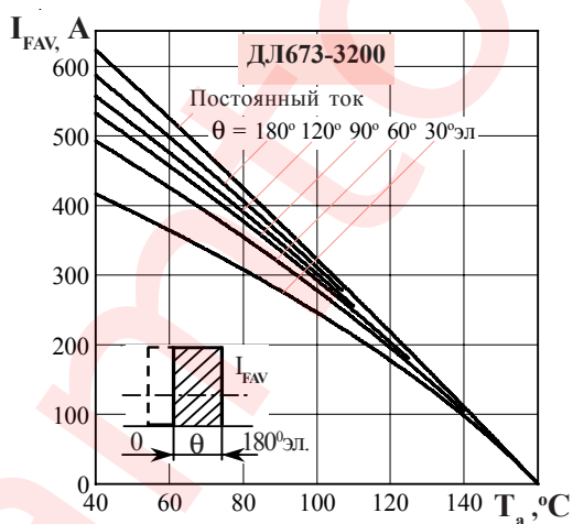
Рисунок 9 - Зависимость допустимого среднего прямого тока I_{FAV} от температуры окружающей среды T_a при естественном охлаждении на охлаждае О173 при различных углах проводимости для токов прямоугольной формы частотой f = 50 Гц и постоянного тока.
