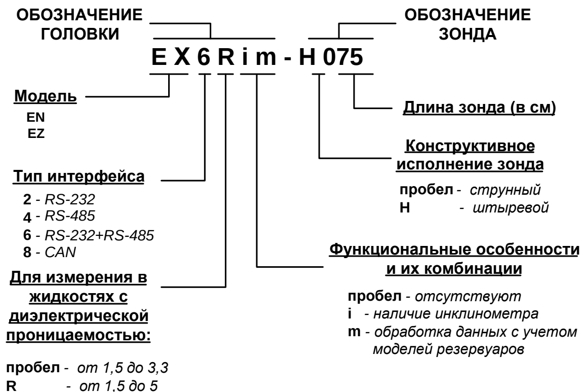
Рис. 1.3 – Обозначение датчиков
