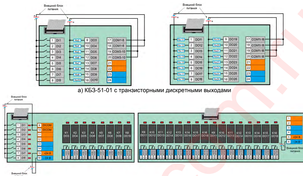
б) КБЗ-44Р-01 с релейными дискретными выходами
