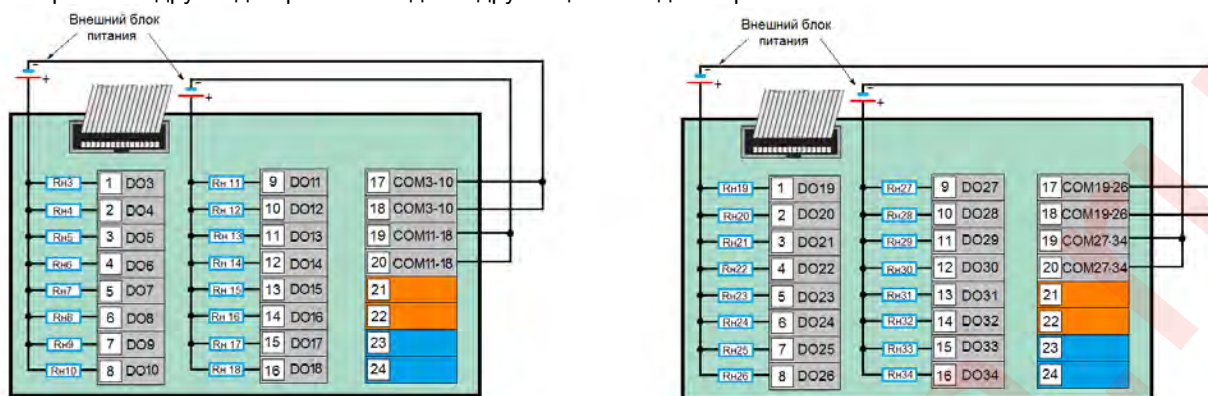
а) КБЗ-51-01 с транзисторными дискретными выходами
