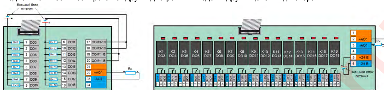
а) KB3-24-20 с транзисторными дискретными выходами
