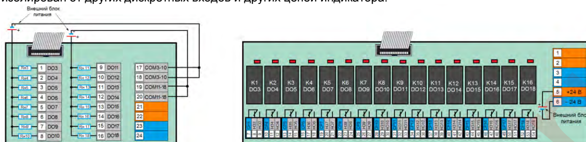
а) КБЗ-24-20 с транзисторными дискретными выходами
