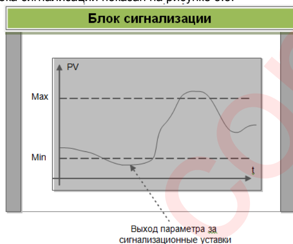
Рисунок 3.5 – Блок-схема блока сигнализации
