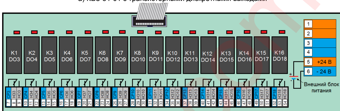
а) КБЗ-51-01 с транзисторными дискретными выходами
