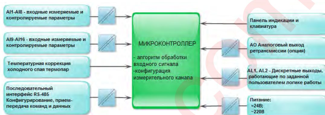
Рисунок 3.2 - Структурная схема индикатора ИТМ-16
