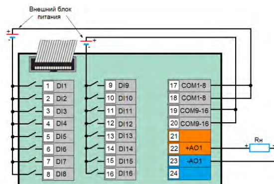
Рисунок Б.4.1 - КБЗ-24-20. Схема подключения сигналов модуля расширения MP-52-11, внешний вид
