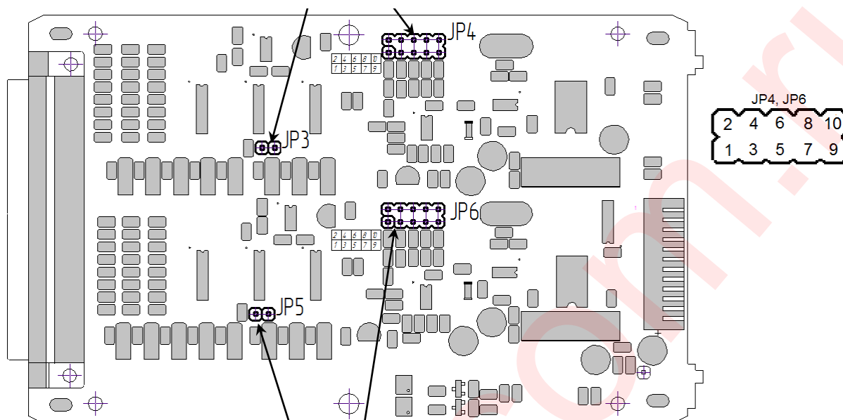
Перемычки 9-16 аналоговых входов
