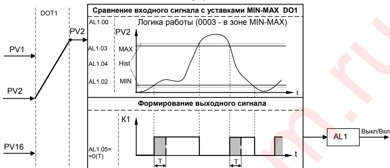
Рисунок 3.6 – Диаграмма работы логических устройств
