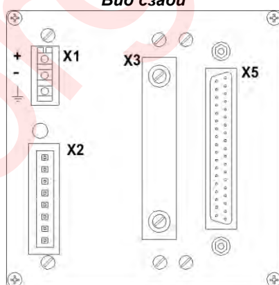
Рисунок А.2 - Габаритные размеры
