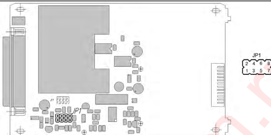
Рисунок 4.5 – Положение перемычек аналогового выхода на модуле расширения.
