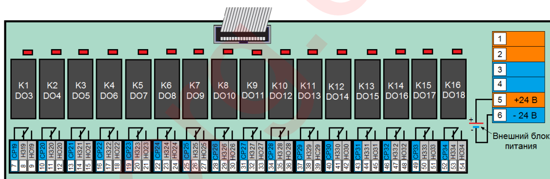
б) КБЗ-55P-01 с релейными дискретными выходами
