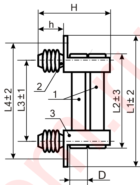
1 – патрон; 2 – изолятор; 3 – контакт. Рис. 6.
