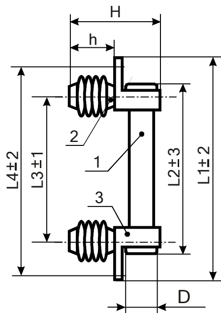
1 – патрон; 2 – изолятор; 3 – контакт. Рис. 5.
