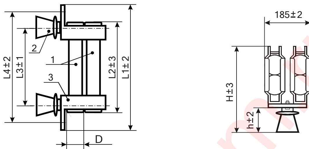
1 – патрон; 2 – изолятор; 3 – контакт. Рис. 7.
