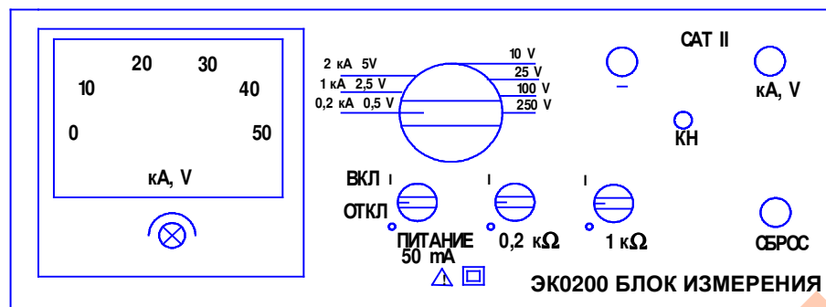
Рисунок 1.1 - Передняя панель блока измерения
