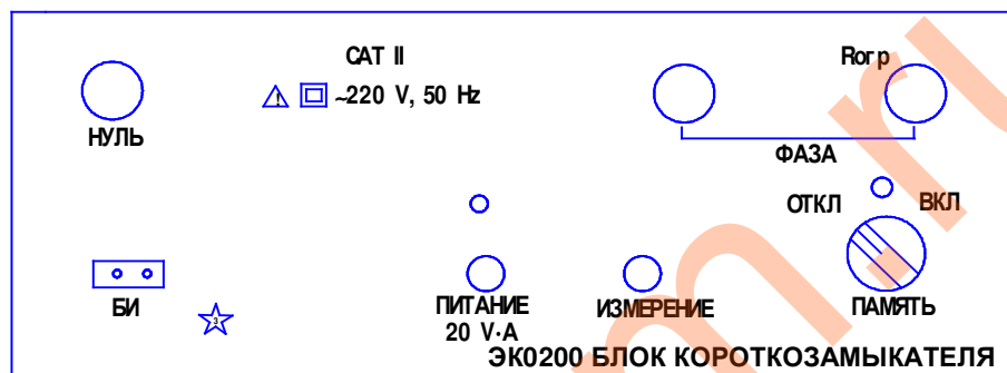
Рисунок 1.2 - Передняя панель блока короткозамыкателя
