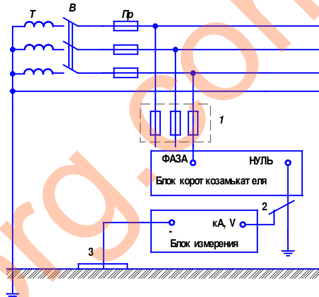
Т - трансформатор; Пр - предохранители; В - трехполюсный выключатель; 1 - силовой распределительный щит; 2 - зануленная металлоконструкция (объект); 3 - измерительная пластина (ведро). Рисунок 2.2 - Измерение напряжения прикосновения
