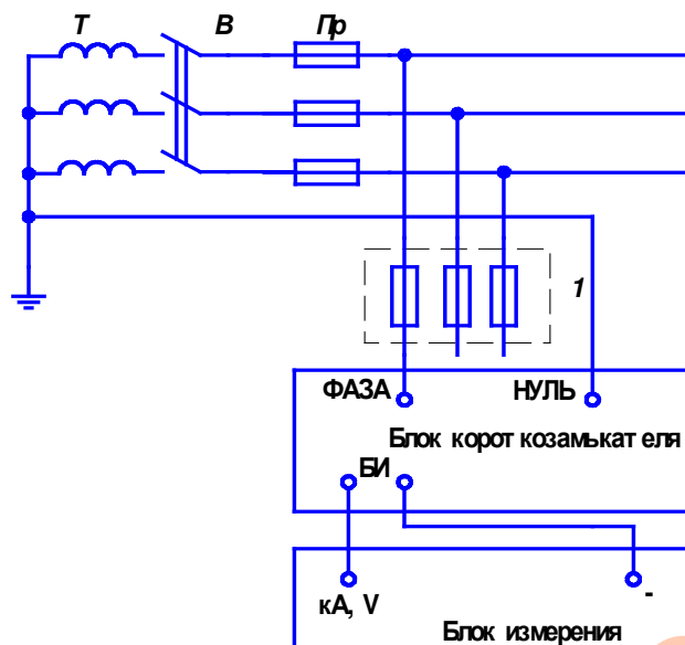
Т - трансформатор; В - трехполюсный выключатель Пр – предохранители; 1 - силовой распределительный щит Рисунок 2.1 - Измерение тока короткого замыкания
