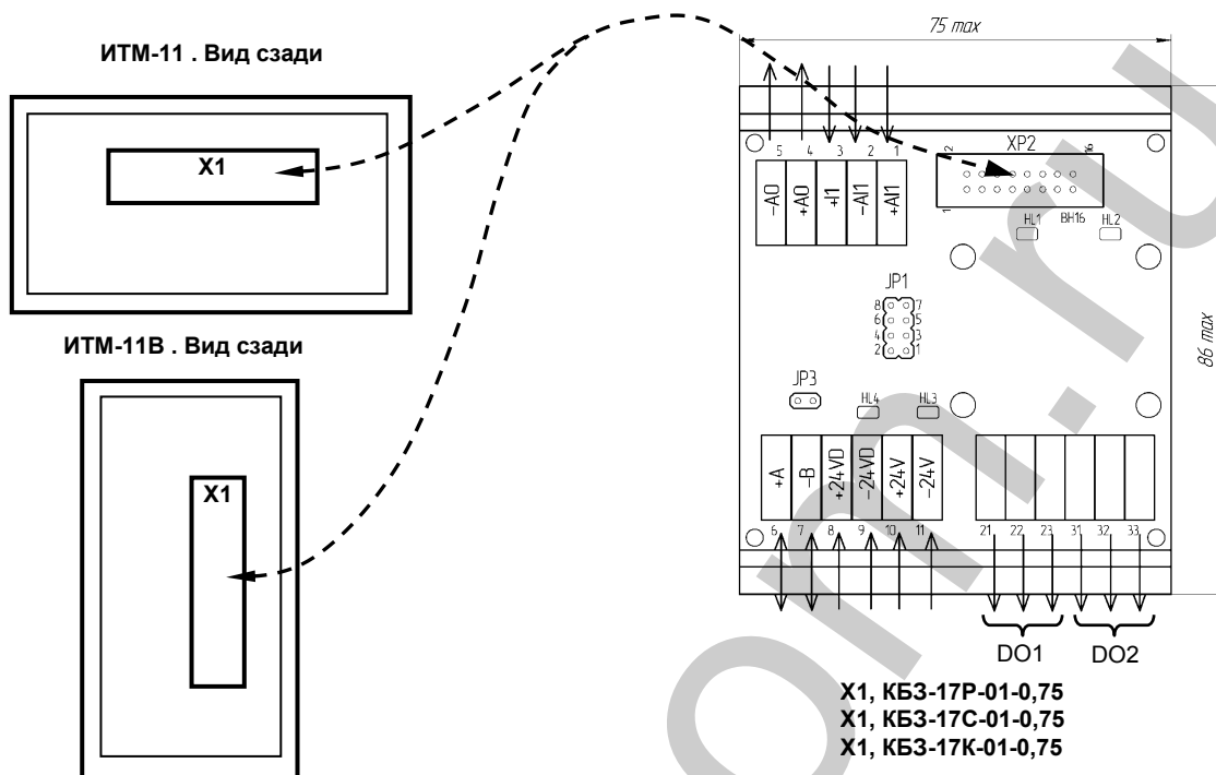
Рисунок Б.2 - Подключение клеммно-блочного соединителя КБЗ-17Р-01-0,75, КБЗ-17С-01-0,75 и КБЗ-17К-01-0,75 к индикатору ИТМ-11, ИТМ-11В
