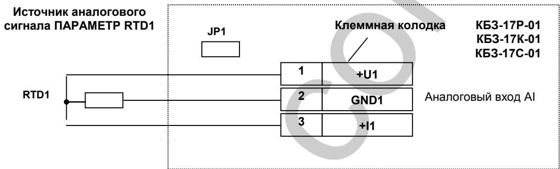
Рисунок Б.10 - Подключение унифицированного аналогового входа индикаторов ИТМ-11, ИТМ-11В
