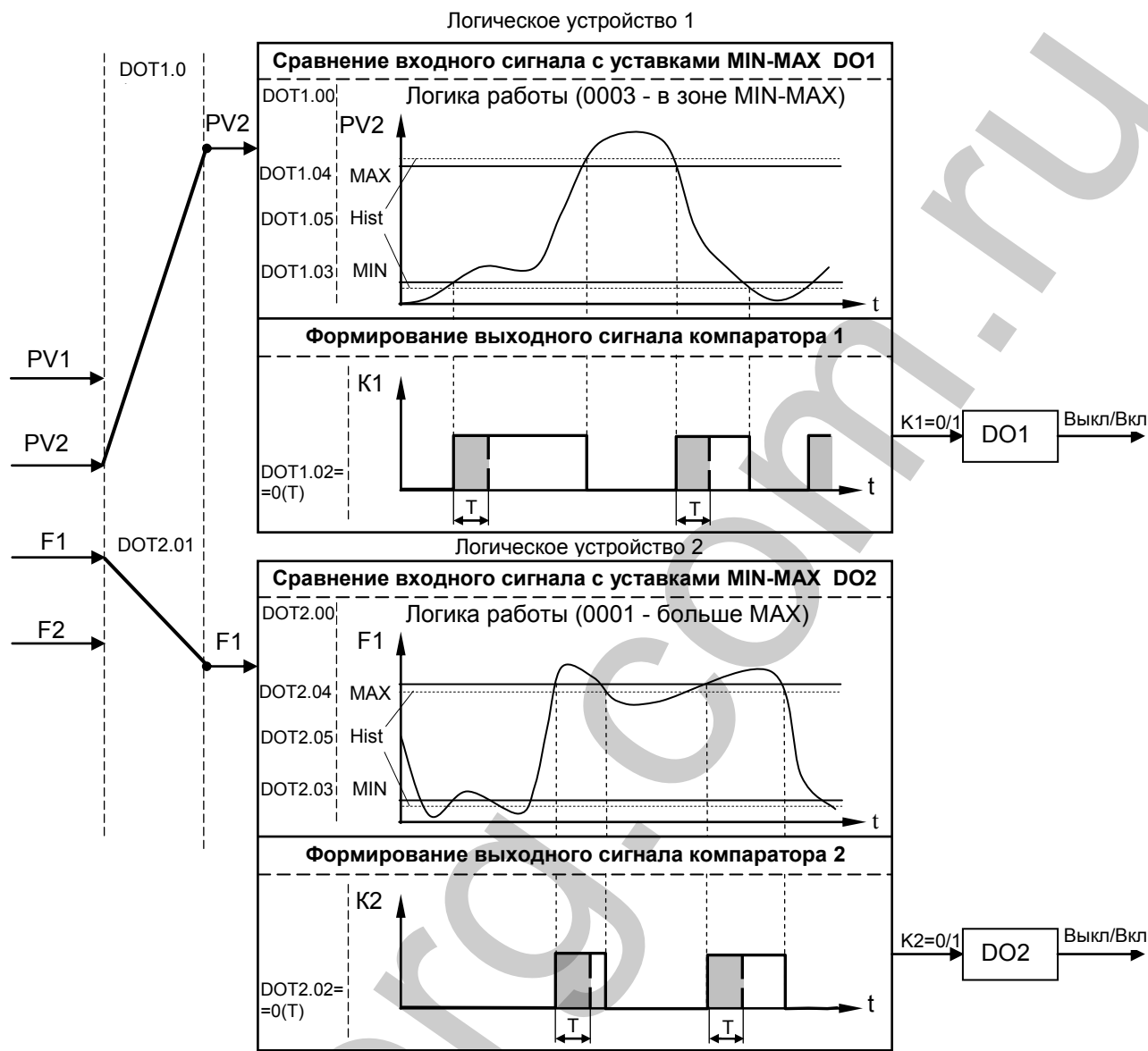
Рисунок 5.9 – Функциональная схема принципа работы компаратора
