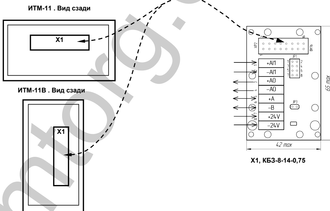
Рисунок Б.3 - Подключение клеммно-блочного соединителя КБЗ-8-14-0,75 к индикаторам ИТМ-11, ИТМ-11В
