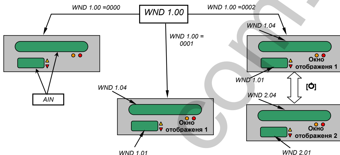
Рисунок 5.7 – Блок-схема выбора вариантов отображения измерительного параметра
