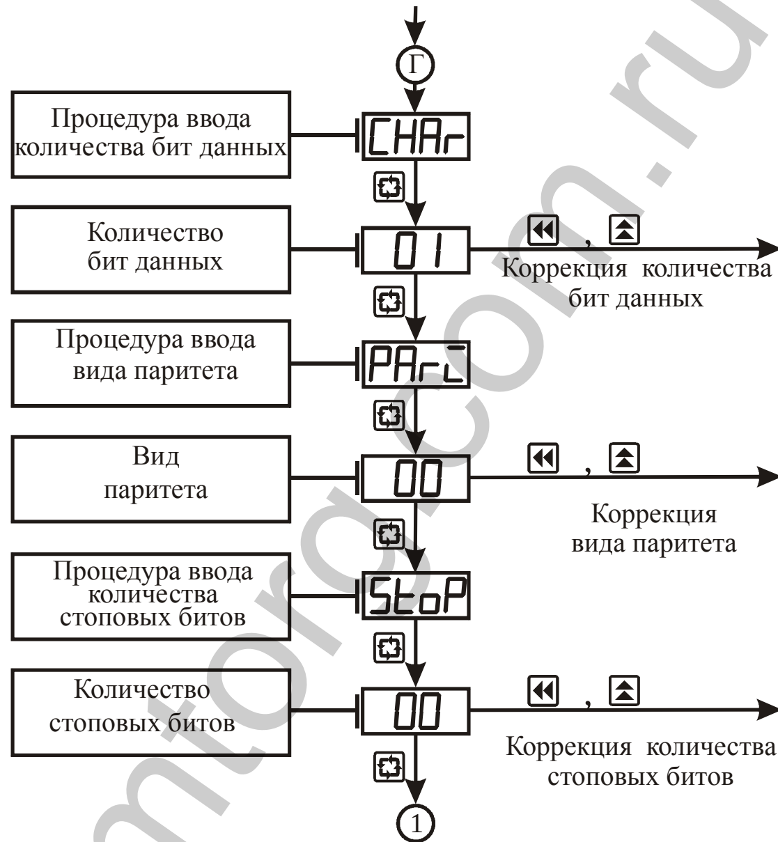
Рисунок 3.12 – Схема алгоритма работы в режиме “Настройка RS” (окончание)
