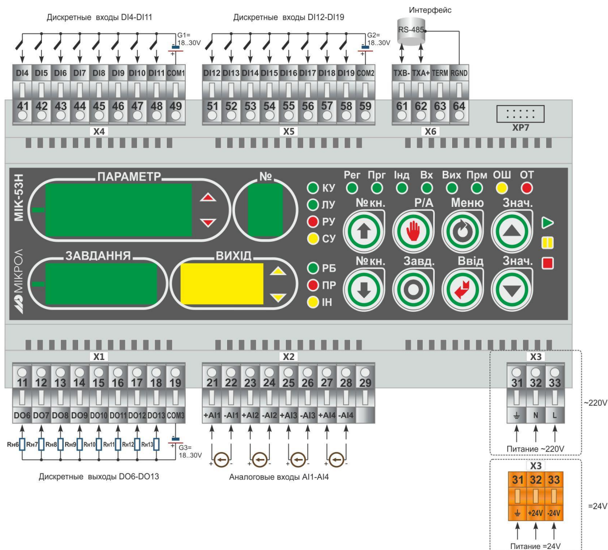
Рисунок 8.8 - Нумерация клемм и сигналы контроллеров МИК-53Н-41
