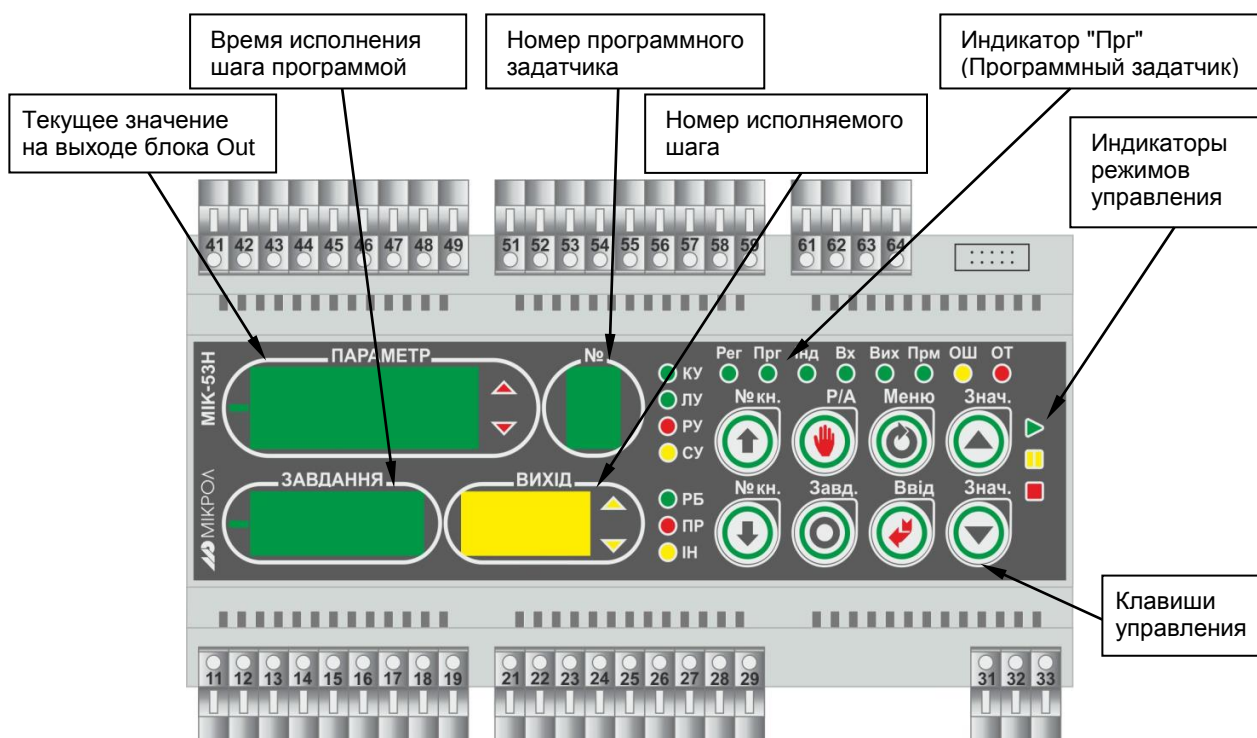
Рисунок 4.4 - Лицевая панель в режиме оперативного управления программным задачиком
