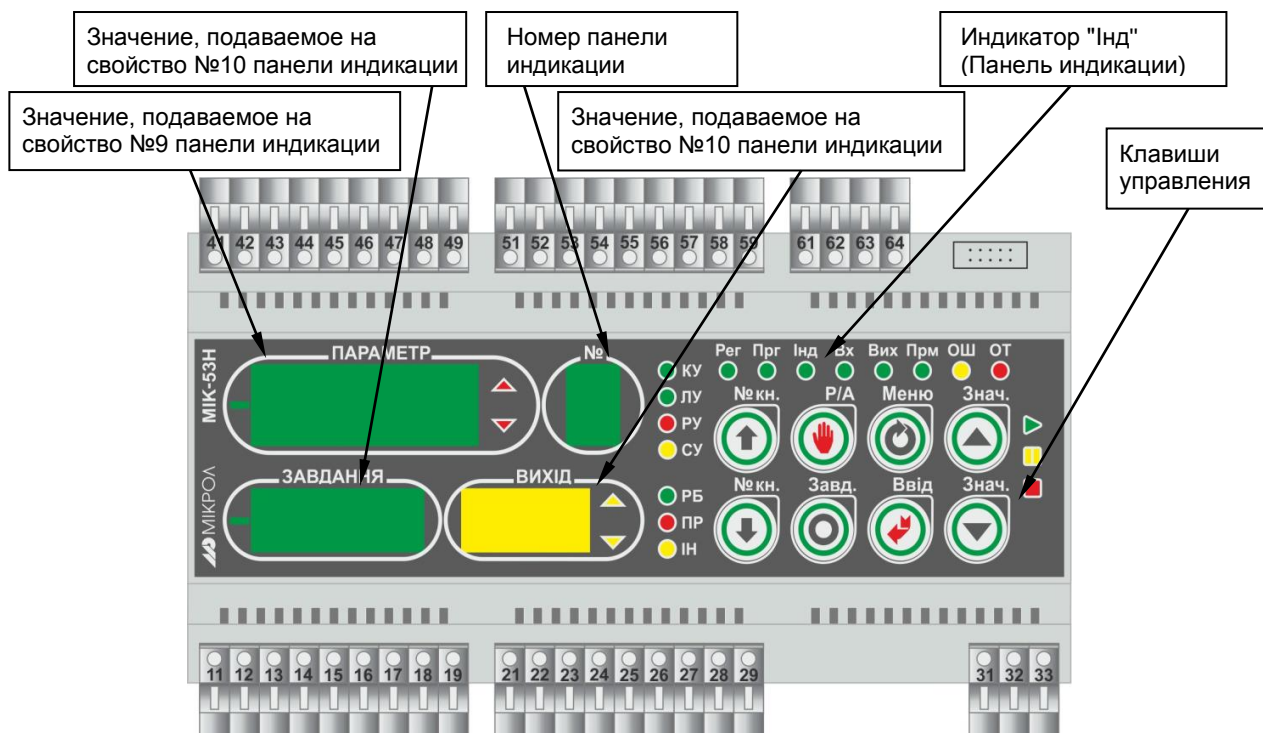
Рисунок 4.5 - Лицевая панель в режиме оперативного управления панелями индикации
