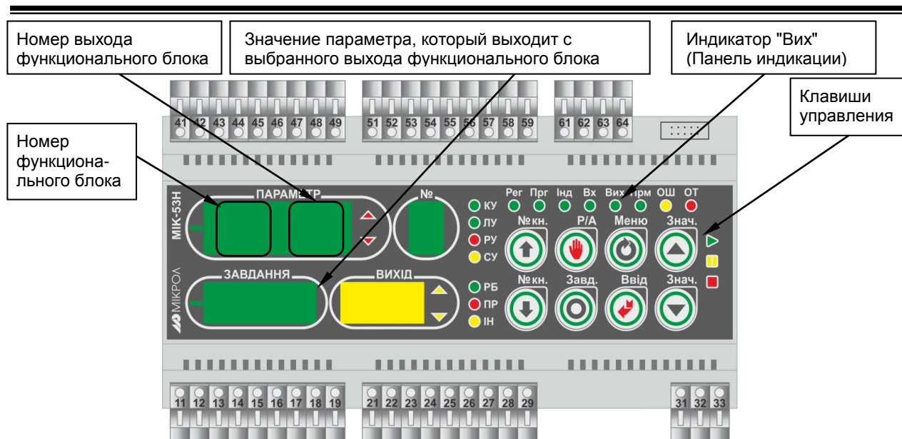
Рисунок 4.7 - Лицевая панель в режиме оперативного управления панелью индикации выходов функциональных блоков
