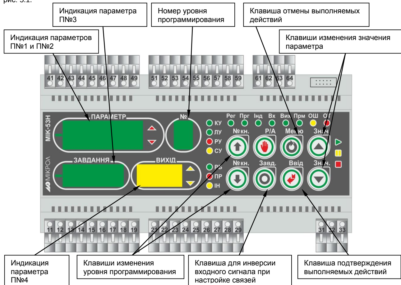
Рисунок 5.1 - Лицевая панель контроллера МИК-53Н в режиме программирования
