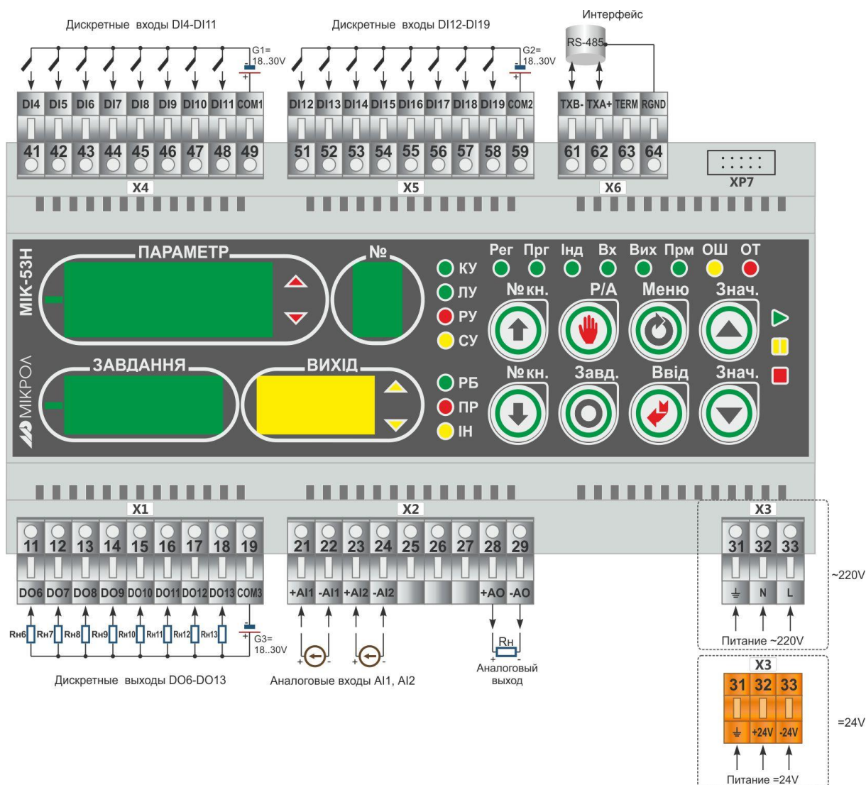
Рисунок 8.3 - Нумерация клемм и сигналы контроллера МИК-53Н-23
