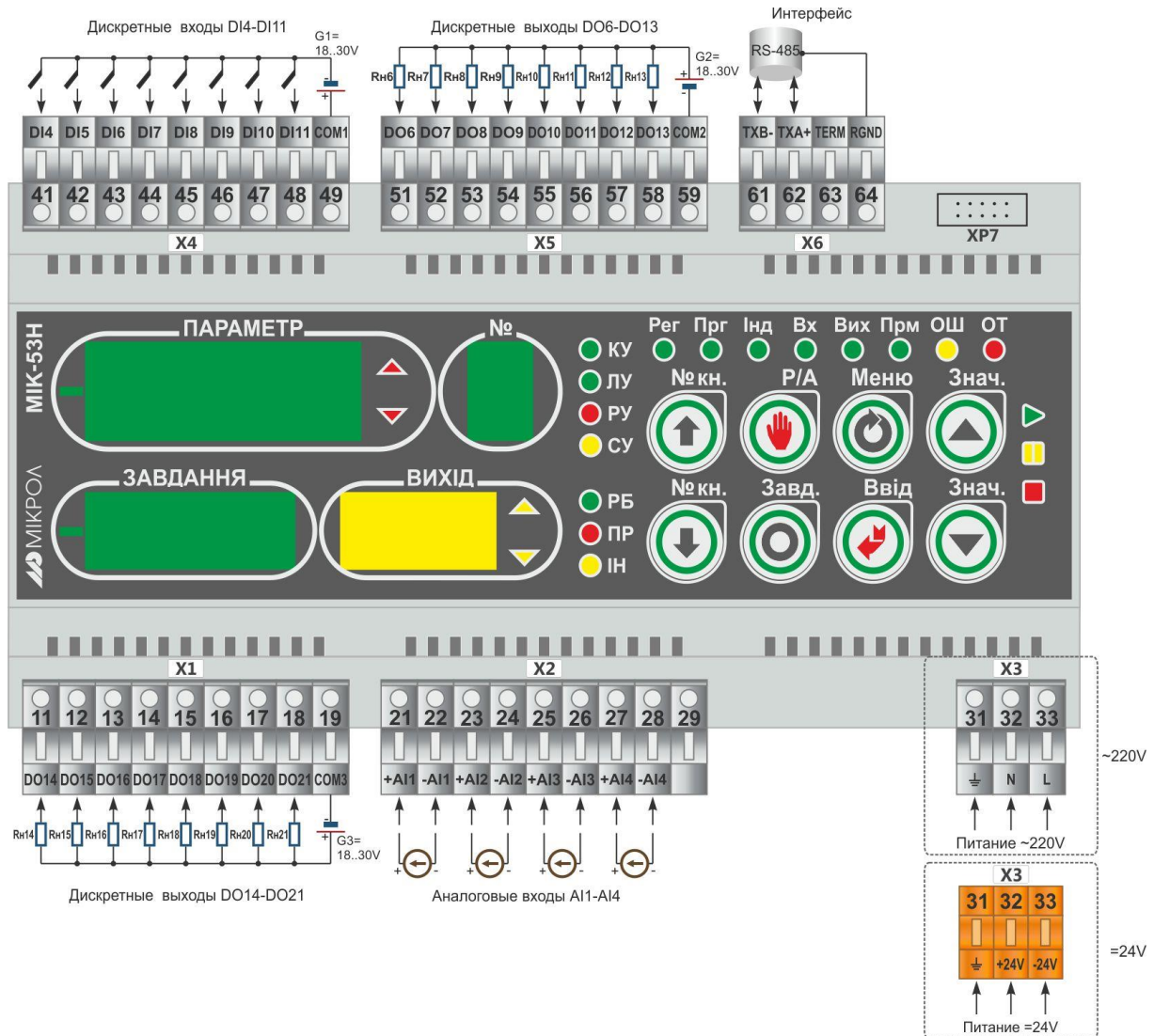
Рисунок 8.9 - Нумерация клемм и сигналы контроллера МИК-53Н-42
