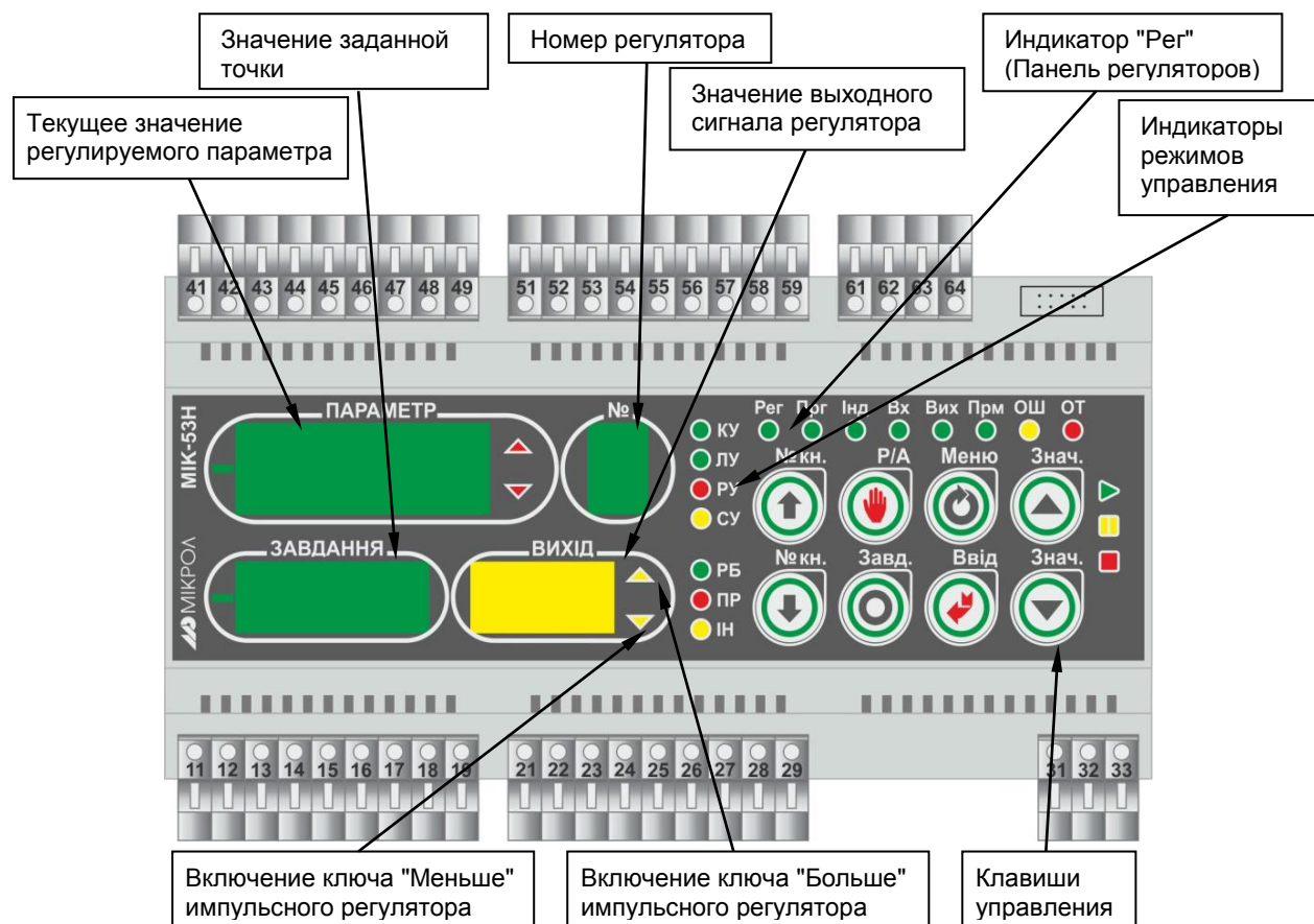
Рисунок 4.3 - Лицевая панель в режиме оперативного управления контурами регулирования
