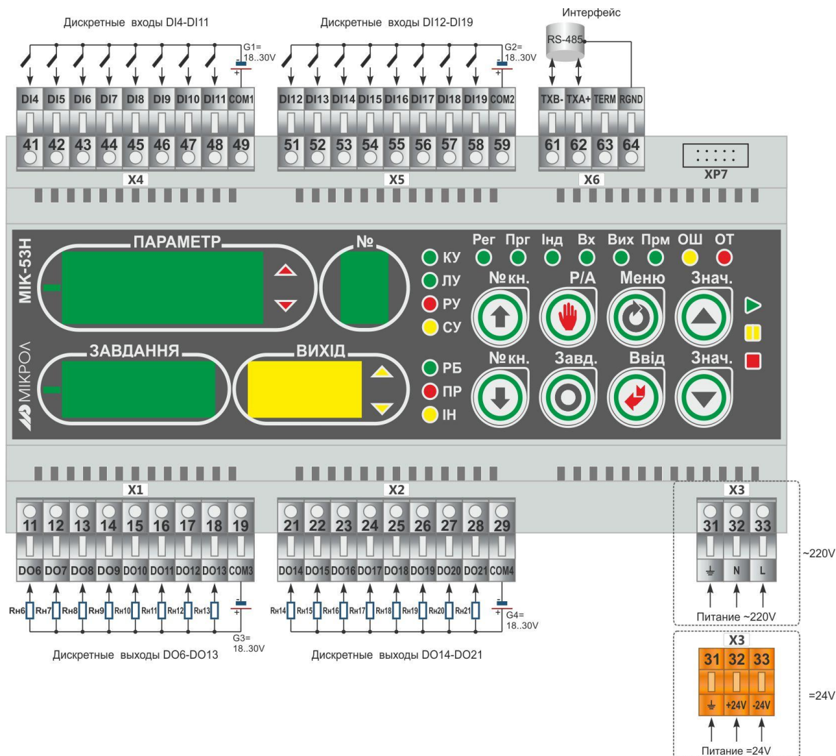
Рисунок 8.6 - Нумерация клемм и сигналы контроллера МИК-53Н-32
