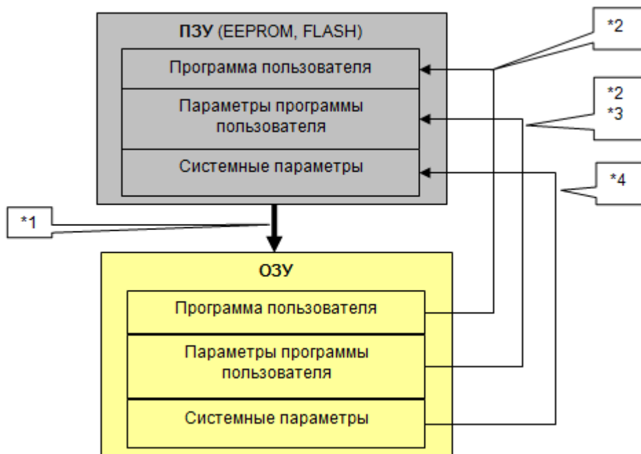
Рисунок 5.4 – Операции копирования и записи программы и параметров между ПЗУ и ОЗУ
