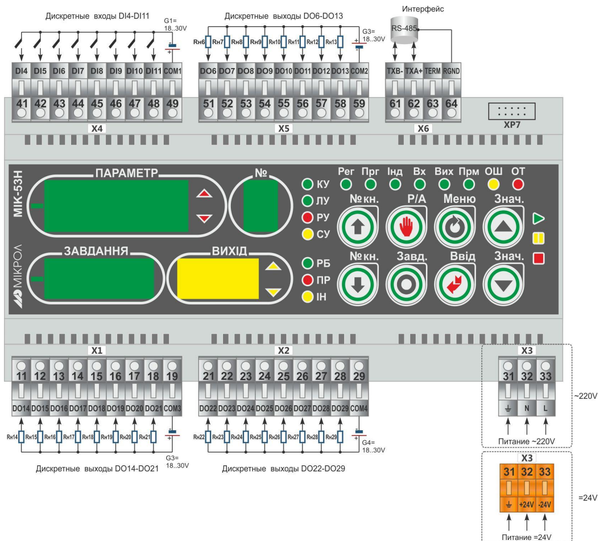
Рисунок 8.7 - Нумерация клемм и сигналы контроллера МИК-53Н-33
