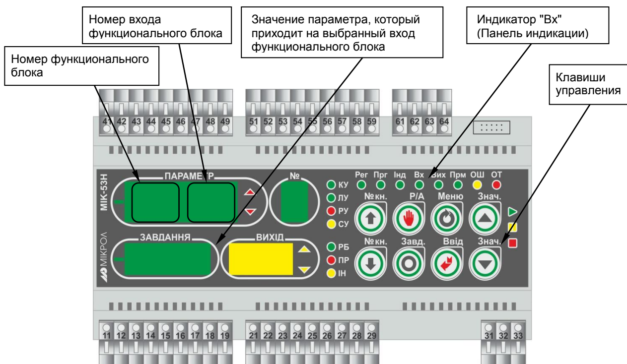
Рисунок 4.6 - Лицевая панель в режиме оперативного управления панелью индикации входов функциональных блоков
