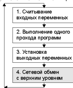
Рисунок 2.9 - Циклограмма работы контроллера
